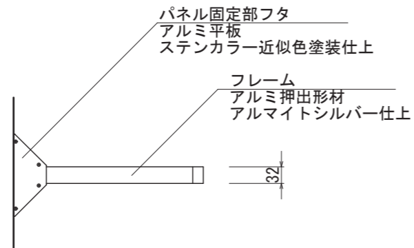
【正面図 S=1:10】
