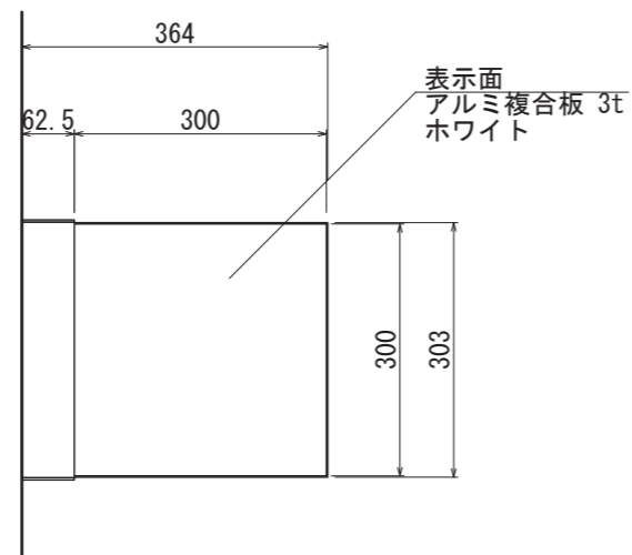
【平面図 S=1:10】
