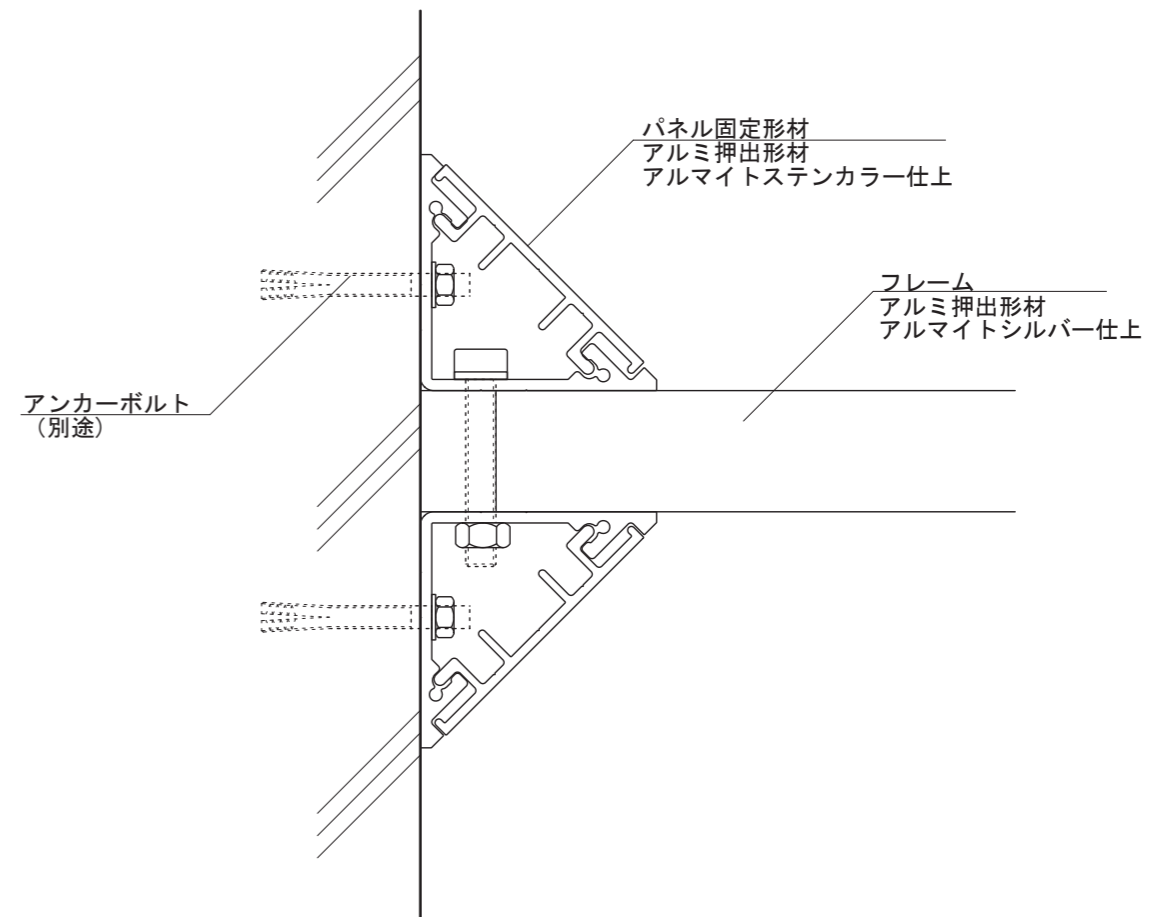
【断面図 S=1:2】
