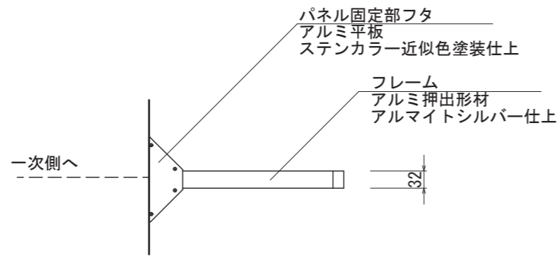
【正面図 S=1:10】
