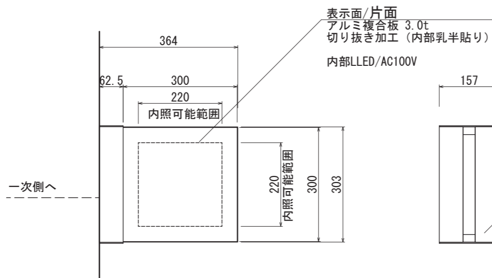
【平面図 S=1:10】
