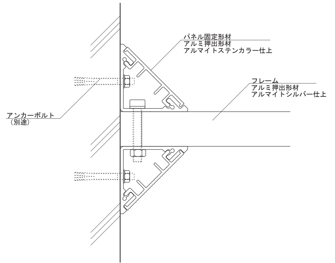
【断面図 S=1:2】
