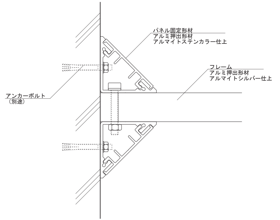
【断面図 S=1:2】
