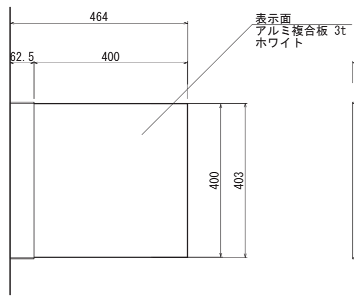
【平面図 S=1:10】
