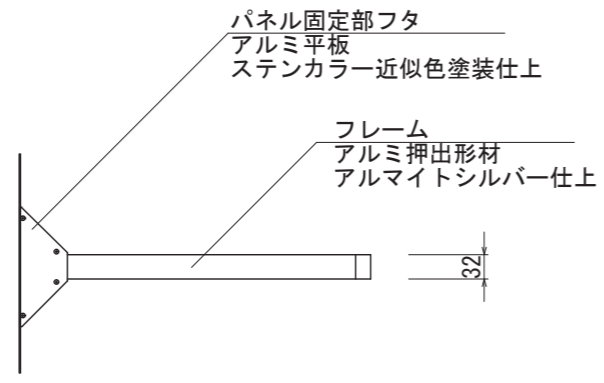
【正面図 S=1:10】
