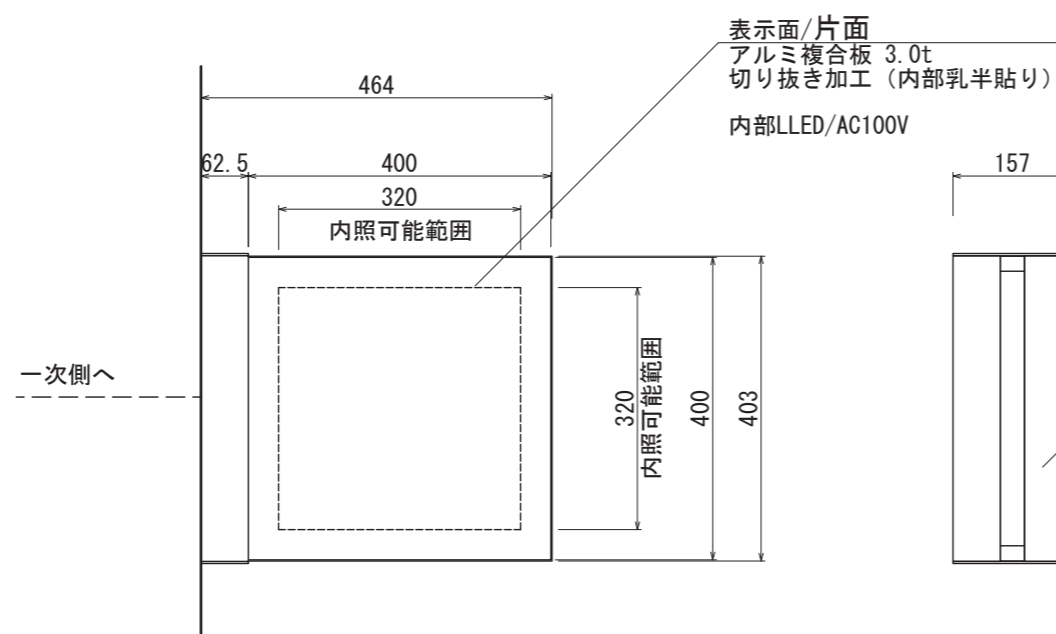
【平面図 S=1:10】
