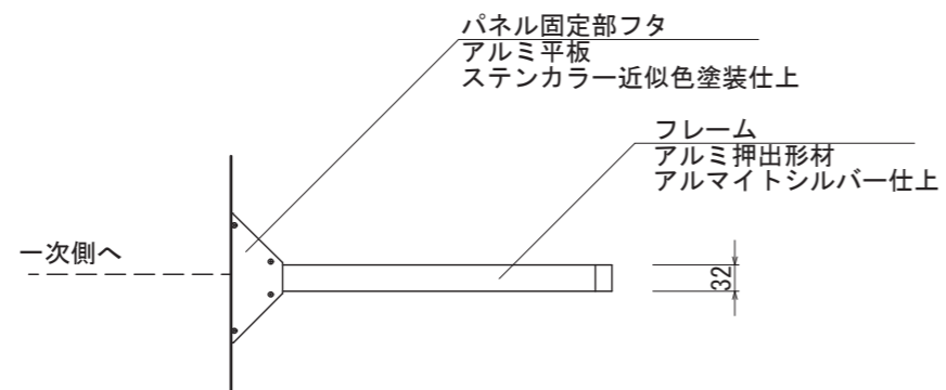
【正面図 S=1:10】
