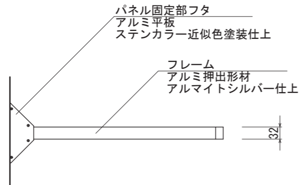
【正面図 S=1:10】
