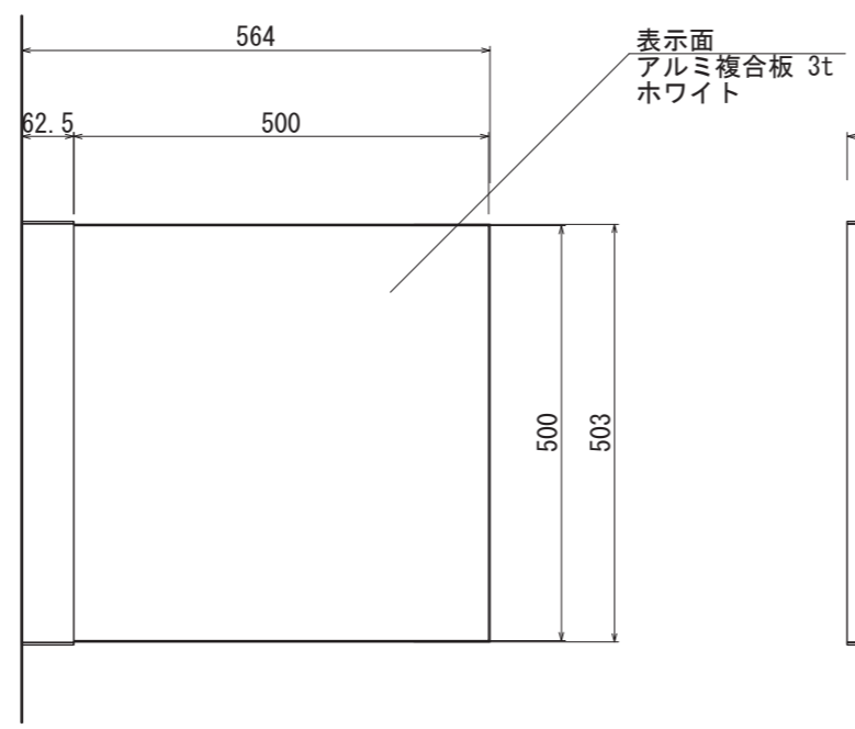
【平面図 S=1:10】
