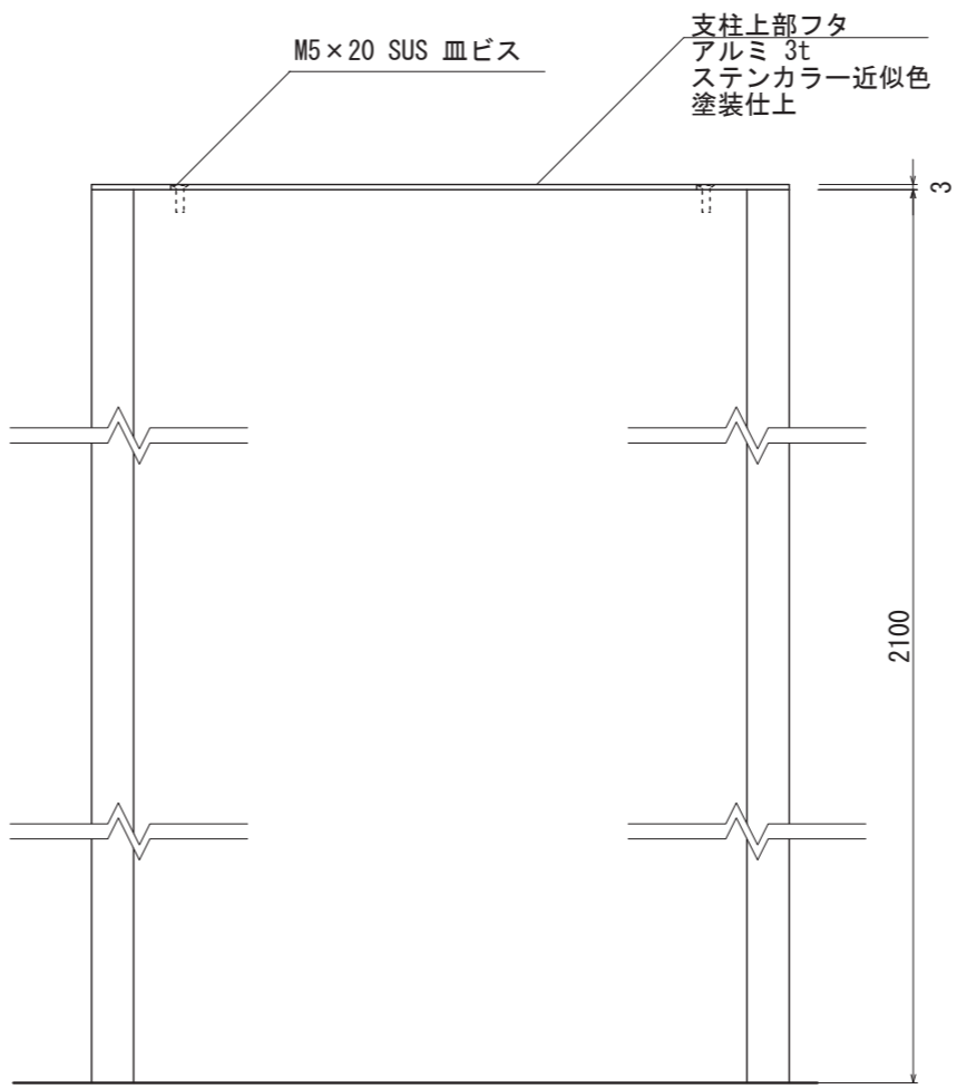
【正面図 S=1:5】
