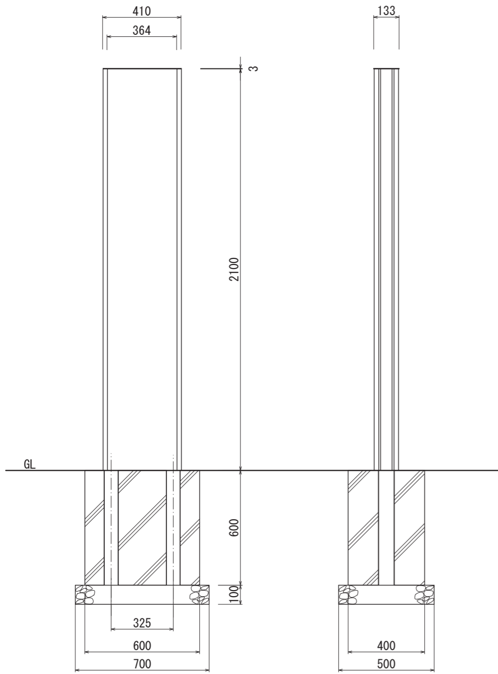
【正面図 S=1:20】
