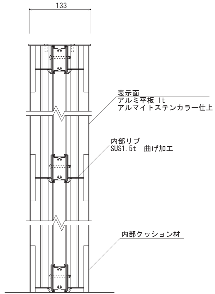
【側断面図 S=1:5】
