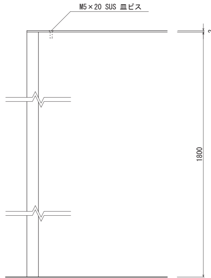
【正面図 S=1:5】
