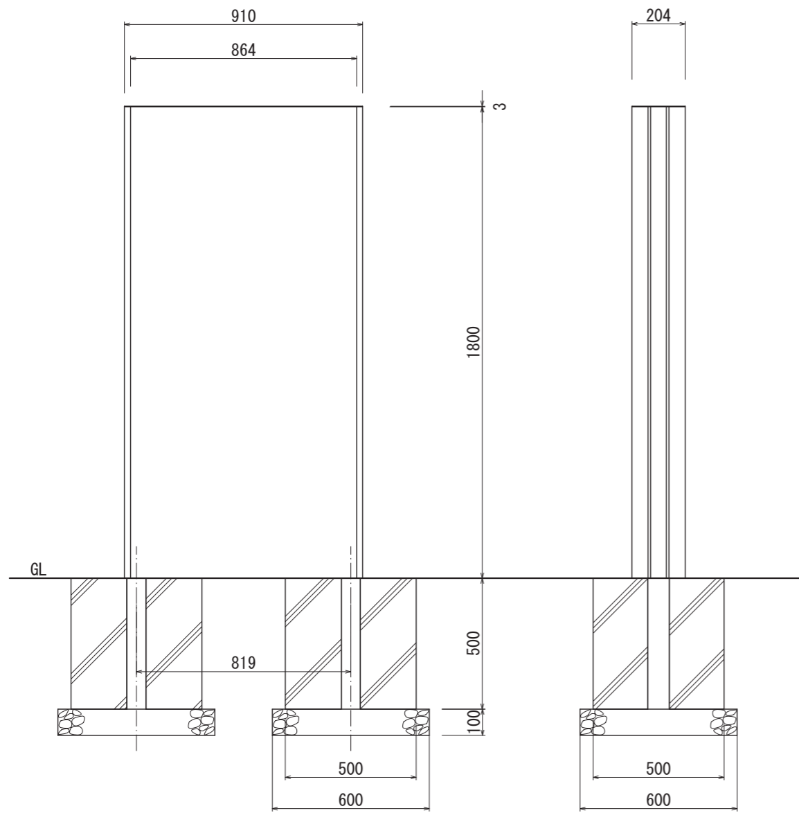
【正面図 S=1:20】
