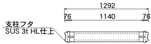
【上面図】
