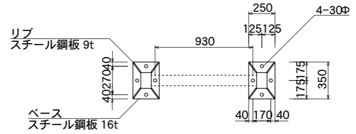
【ベース詳細図】
