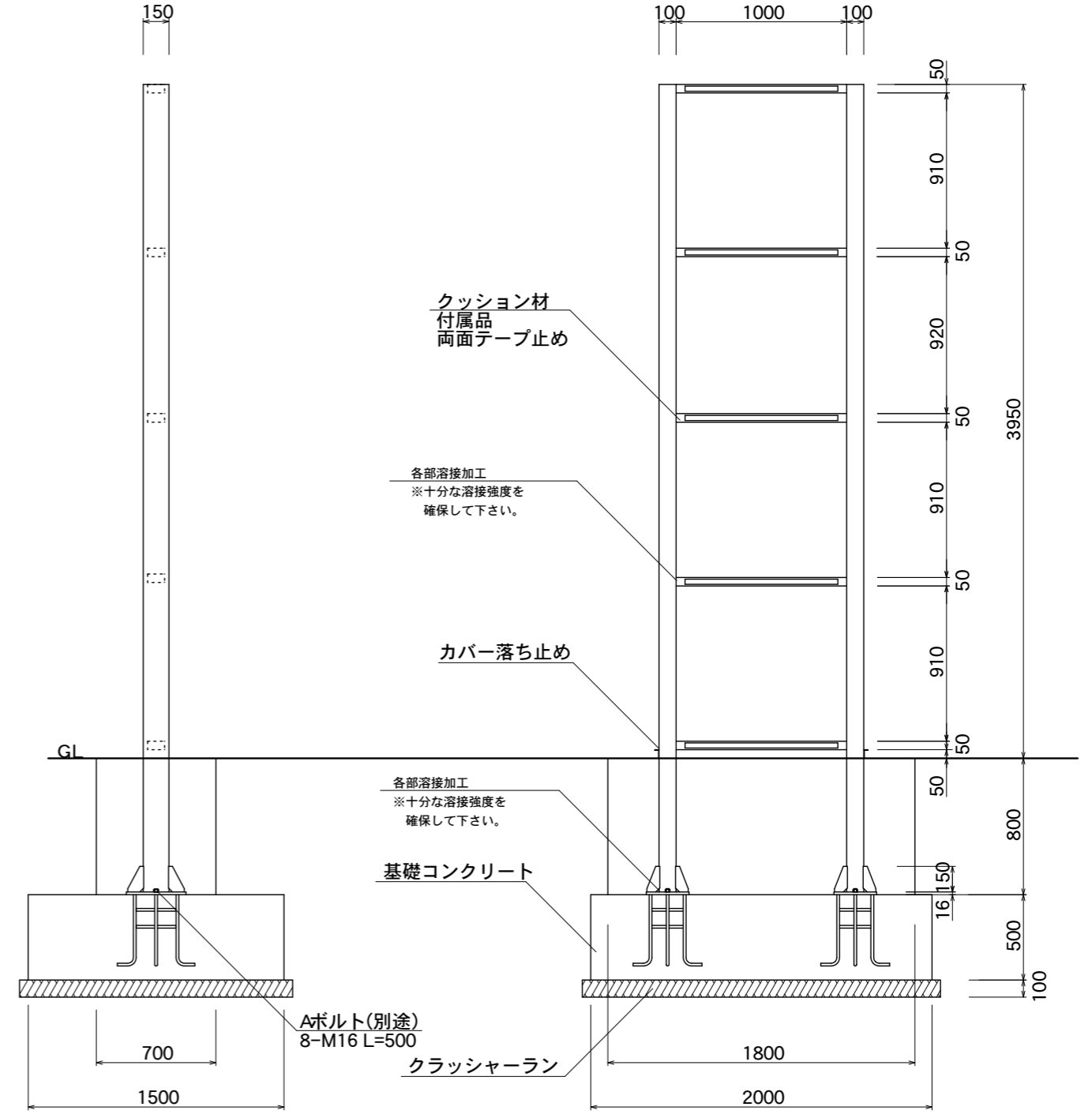
【内部鉄骨断面図】
