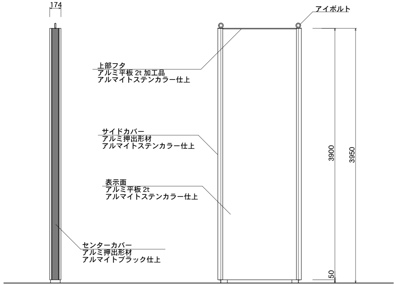
【外観側面図】
