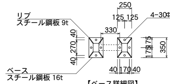
【ベース詳細図】
