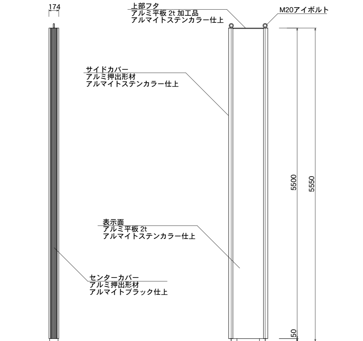
【外観側面図】
