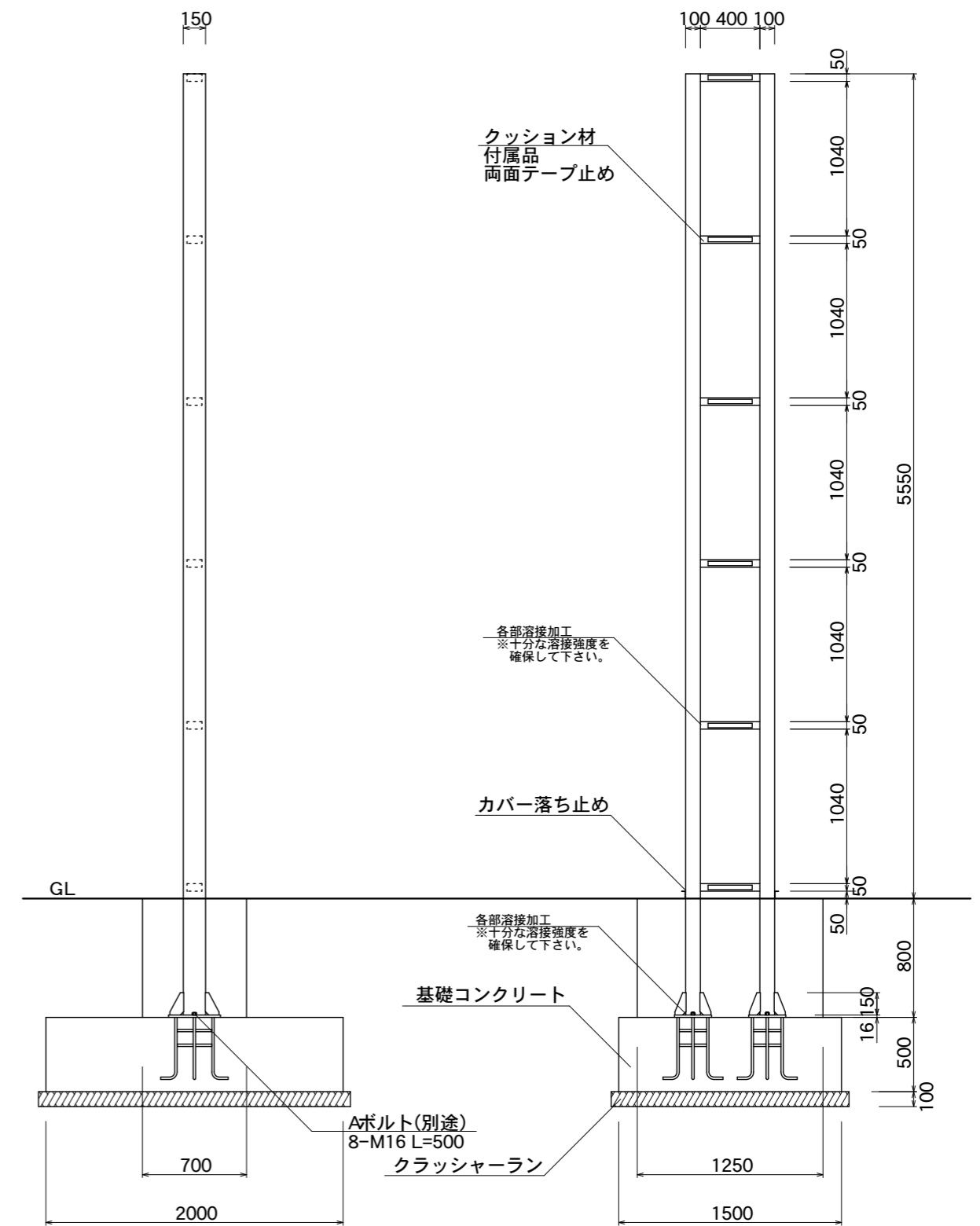
【内部鉄骨断面図】
