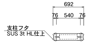
【上面図】
