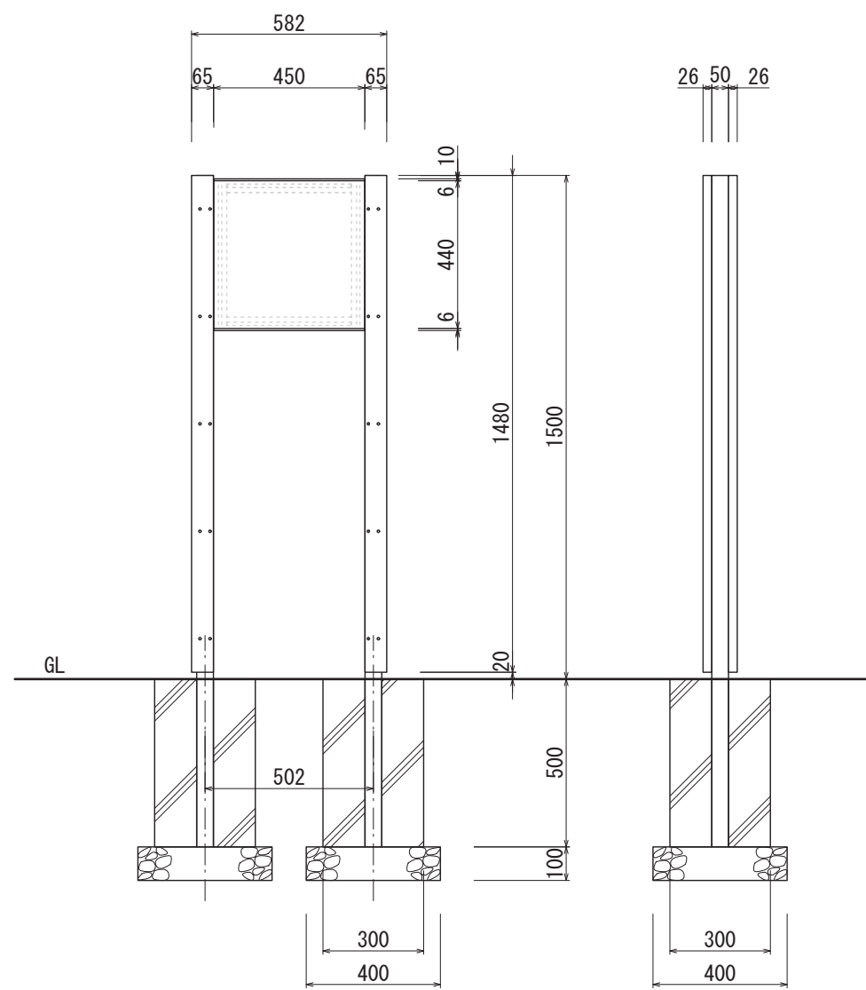
【正面図 S=1:20】
