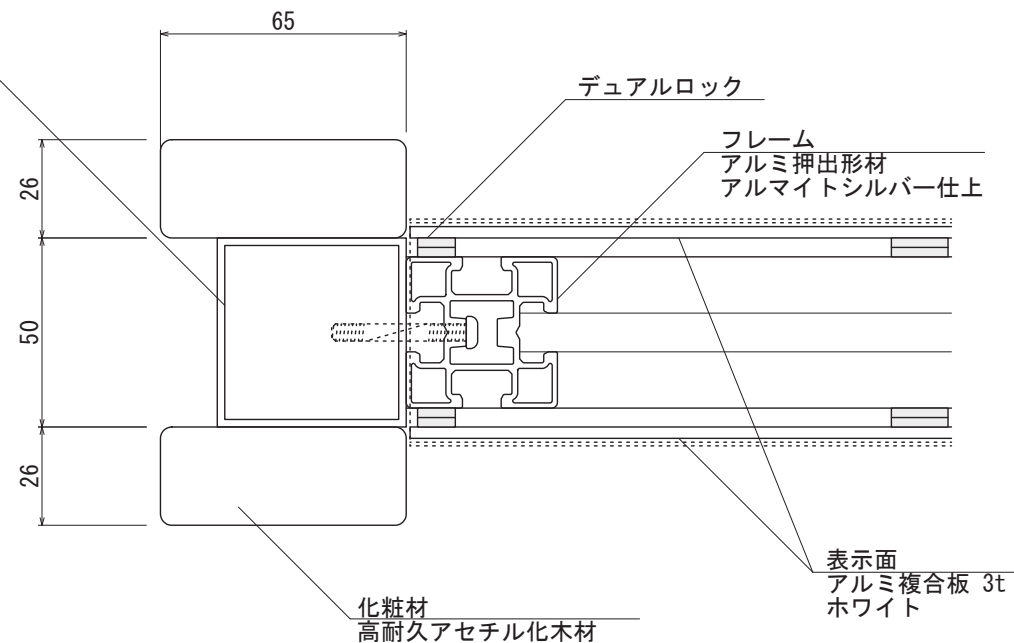
【断面図 S=1:2】
