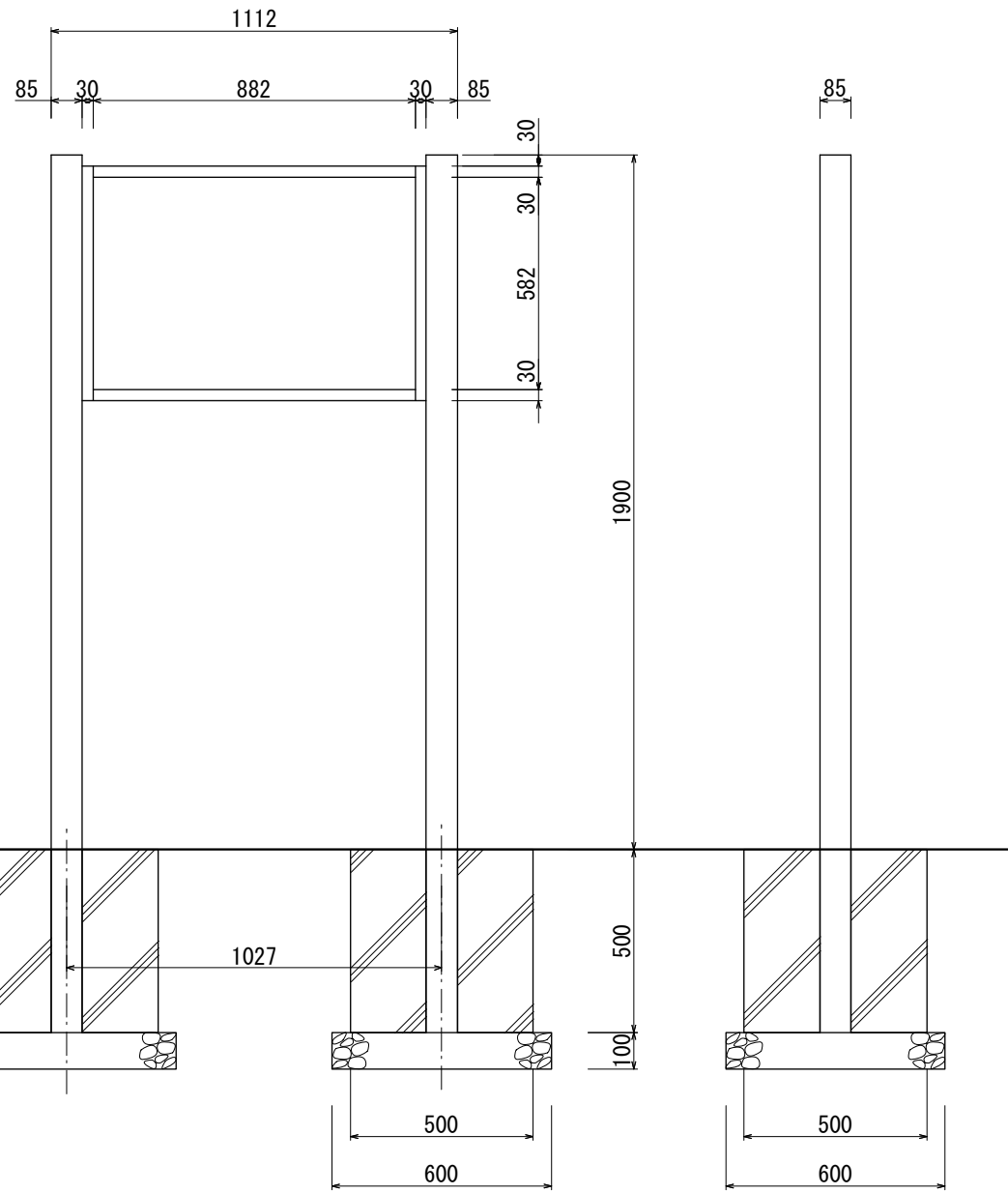
【正面図 S=1:20】
