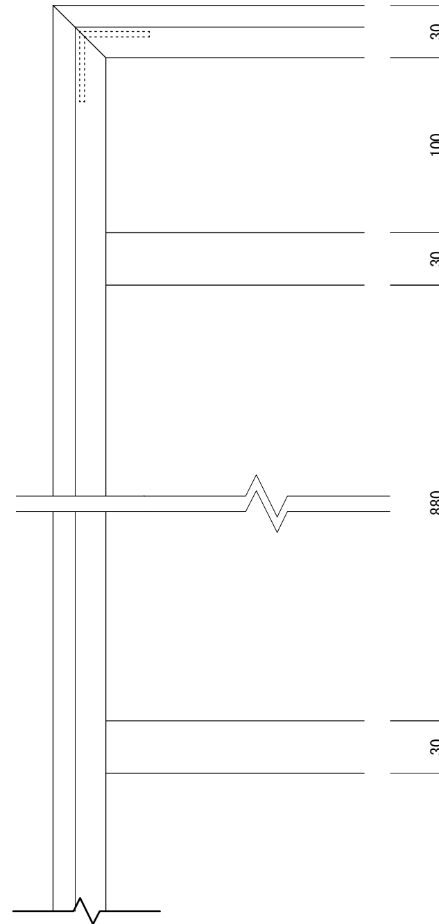
【正面図 S=1:3】
