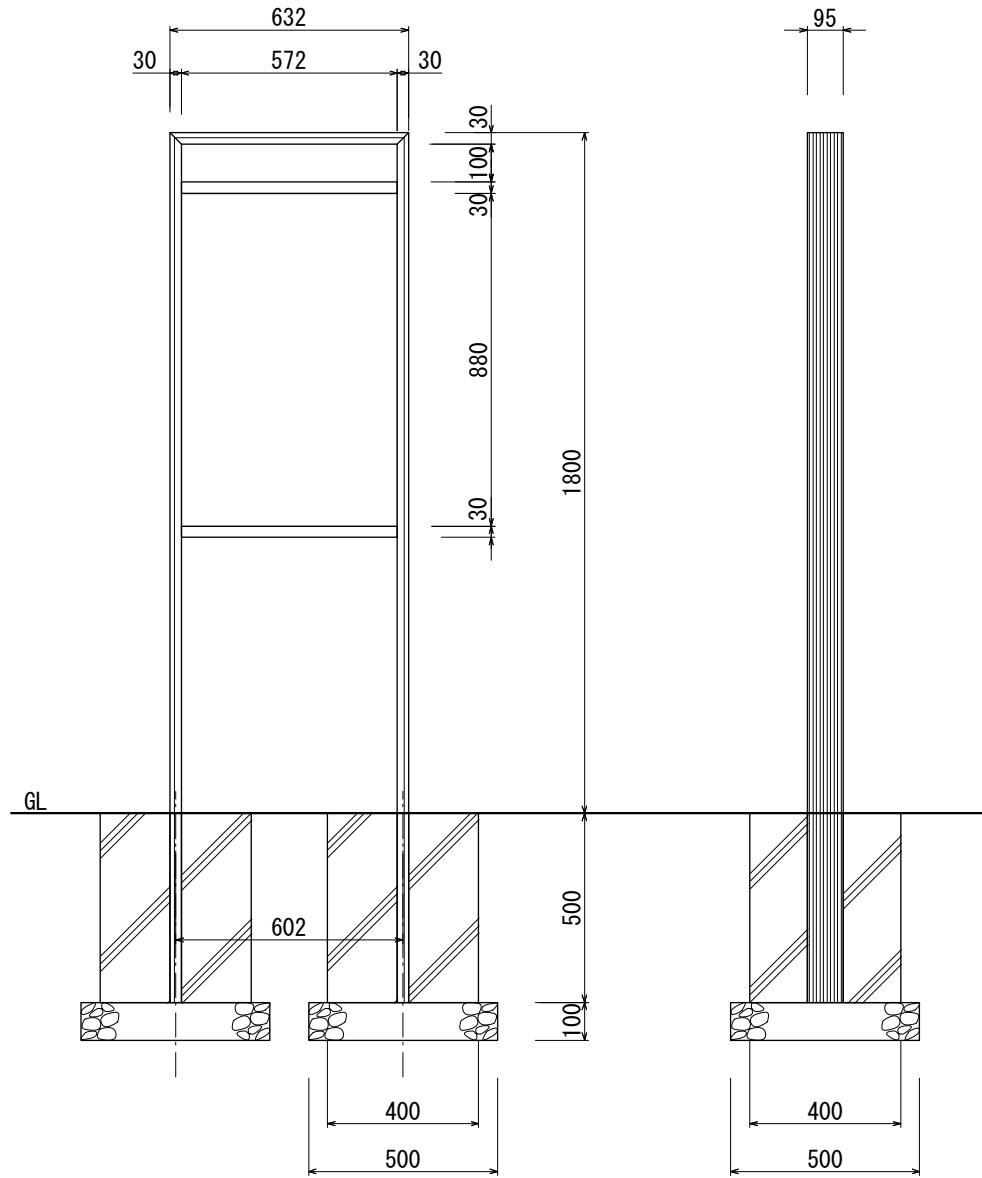
【正面図 S=1:20】
