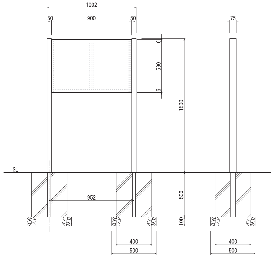
【正面図 S=1:20】
