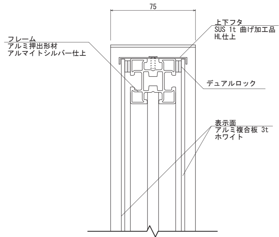
【断面図 S=1:2】
