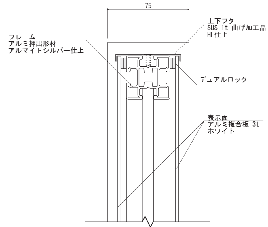
【断面図 S=1:2】
