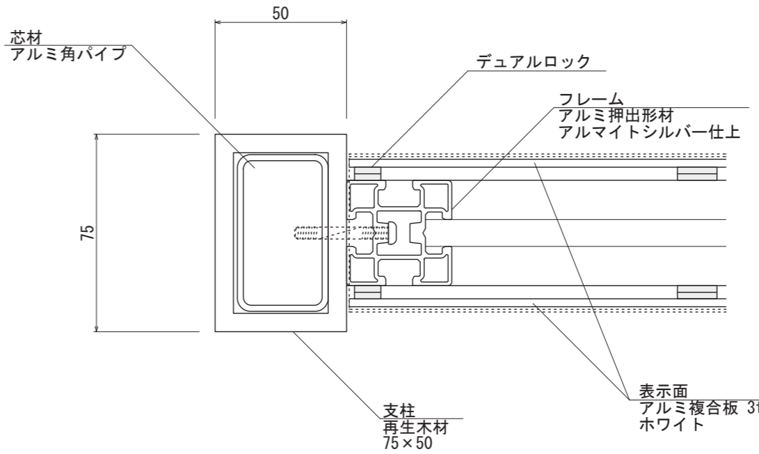
【断面図 S=1:2】
