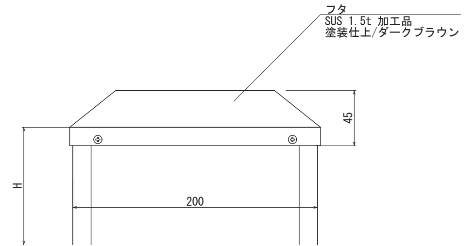
【正面図 S=1:3】
