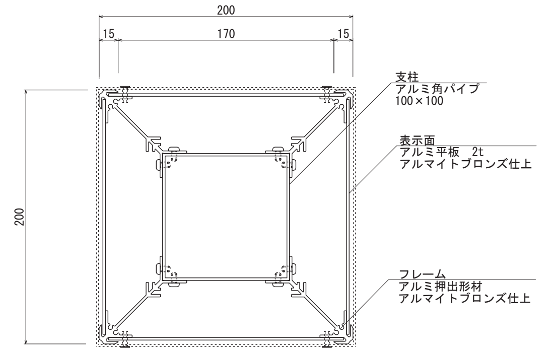
【断面図 S=1:3】
