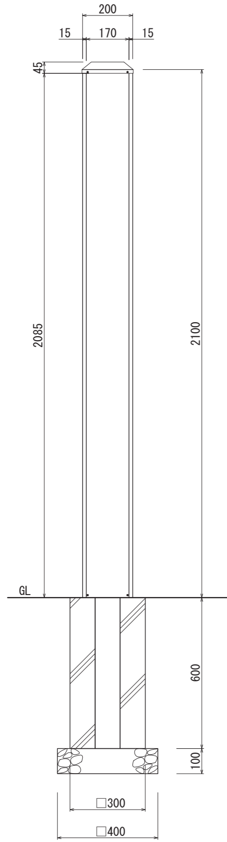
【基礎タイプ】 【正面図 S=1:15】
