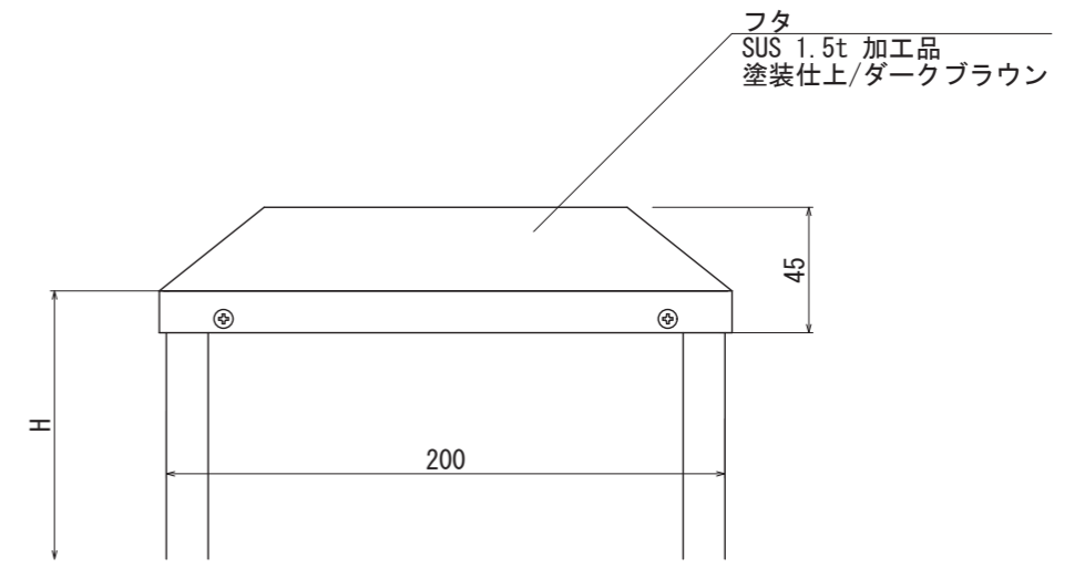
【正面図 S=1:3】
