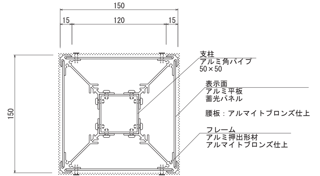
【断面図 S=1:3】
