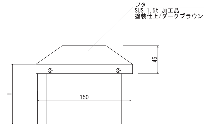
【正面図 S=1:3】
