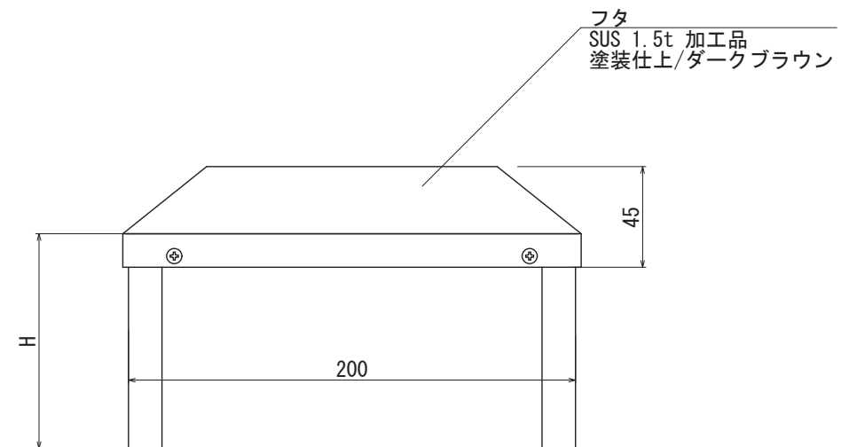
【正面図 S=1:3】
