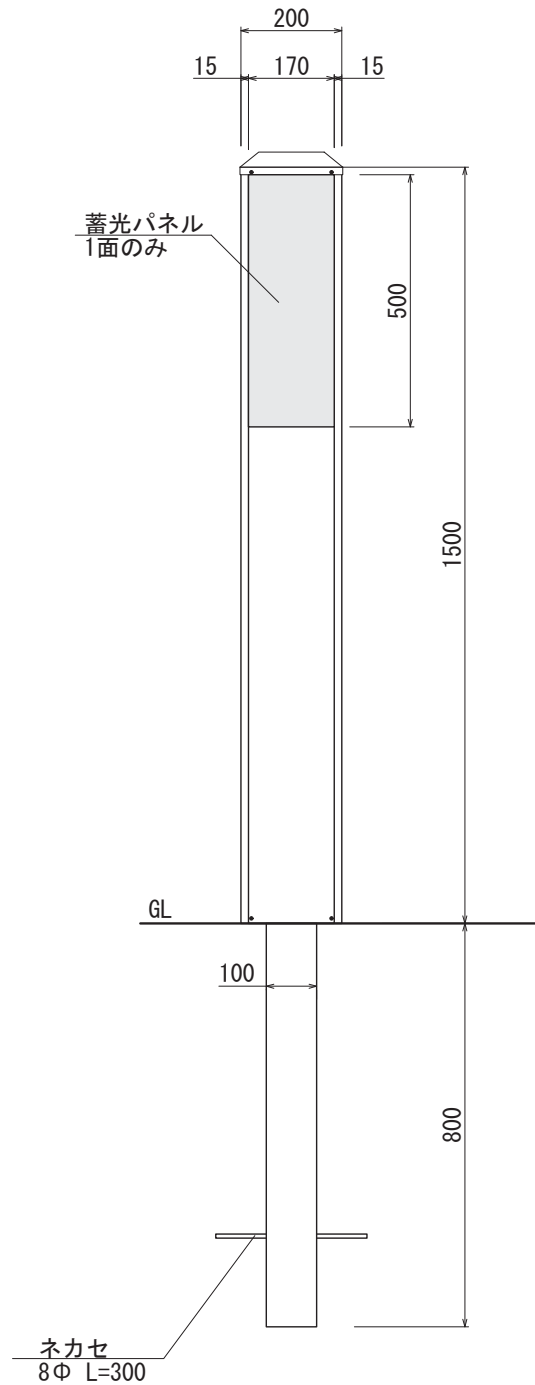
【土中タイプ】
