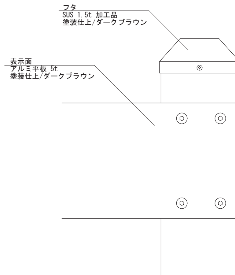
【正面図 S=1:3】
