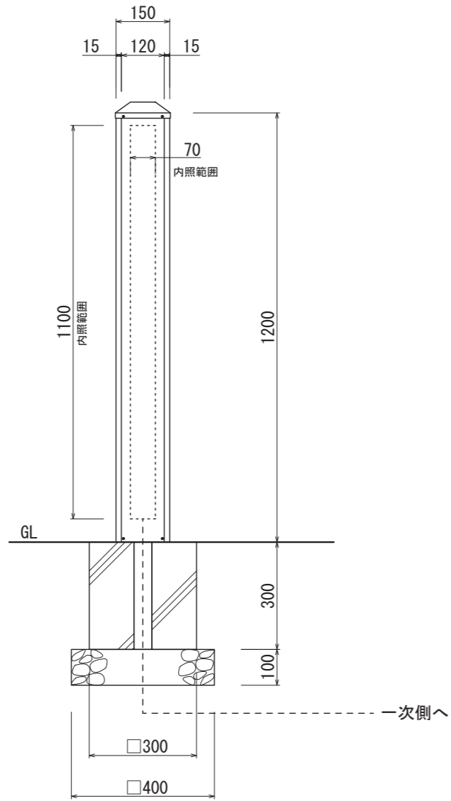
【正面図 S=1:15】
