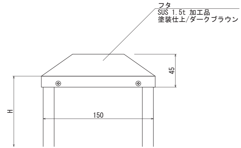
【正面図 S=1:3】
