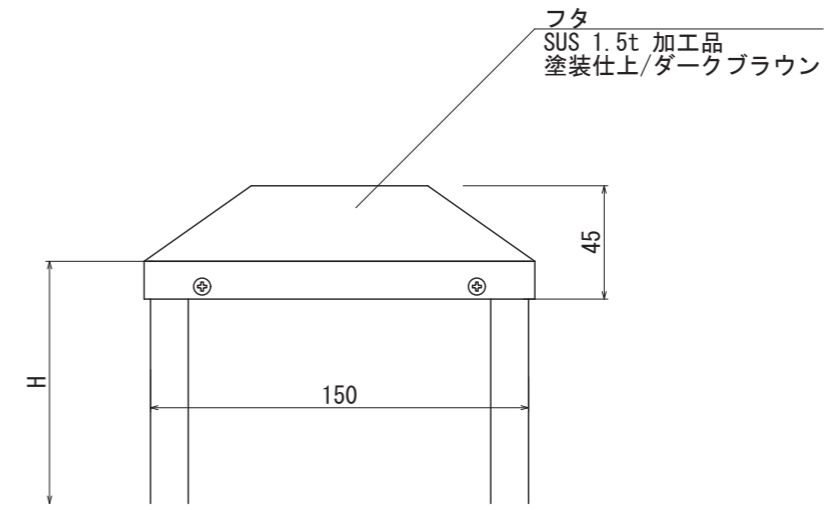
【正面図 S=1:3】
