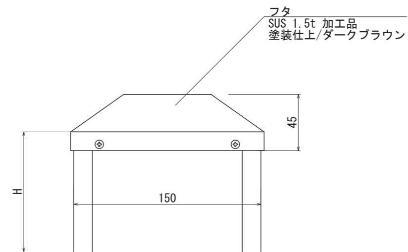
【正面図 S=1:3】
