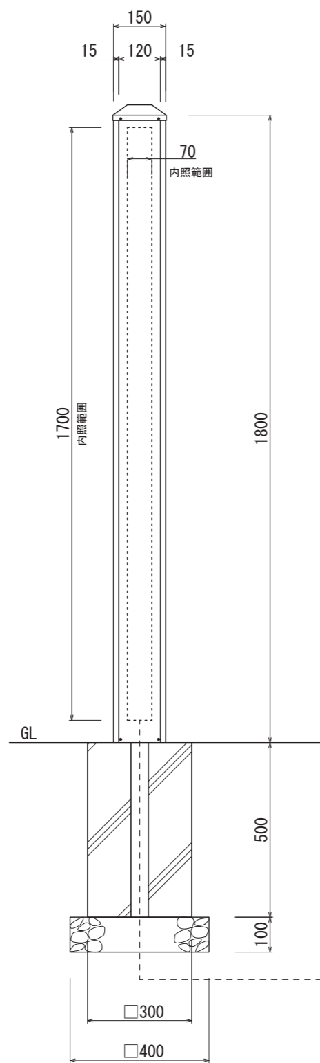
【正面図 S=1:15】
