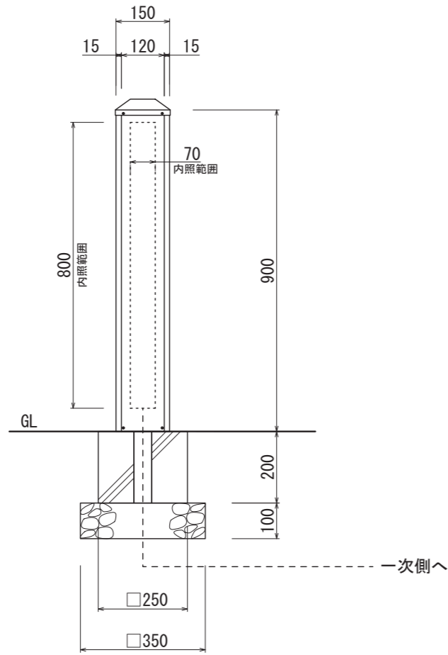
【正面図 S=1:15】
