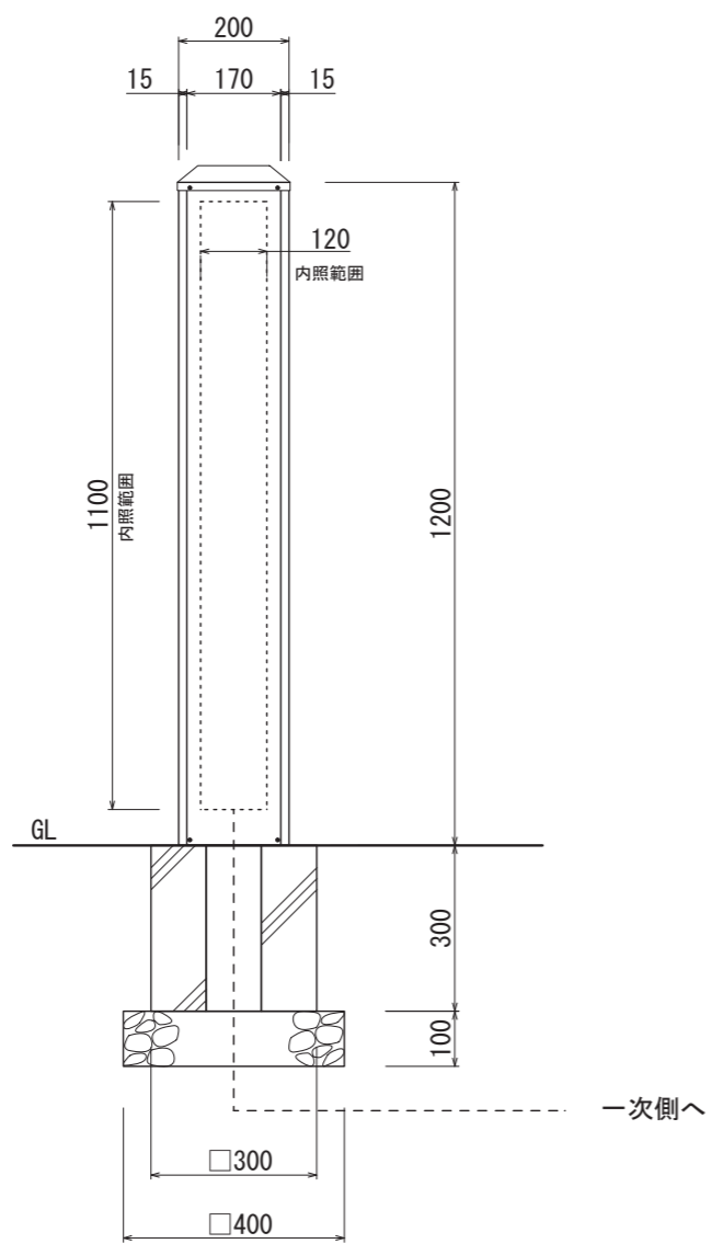
【正面図 S=1:15】
