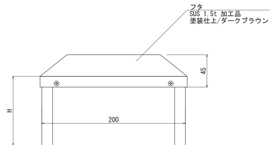
【正面図 S=1:3】
