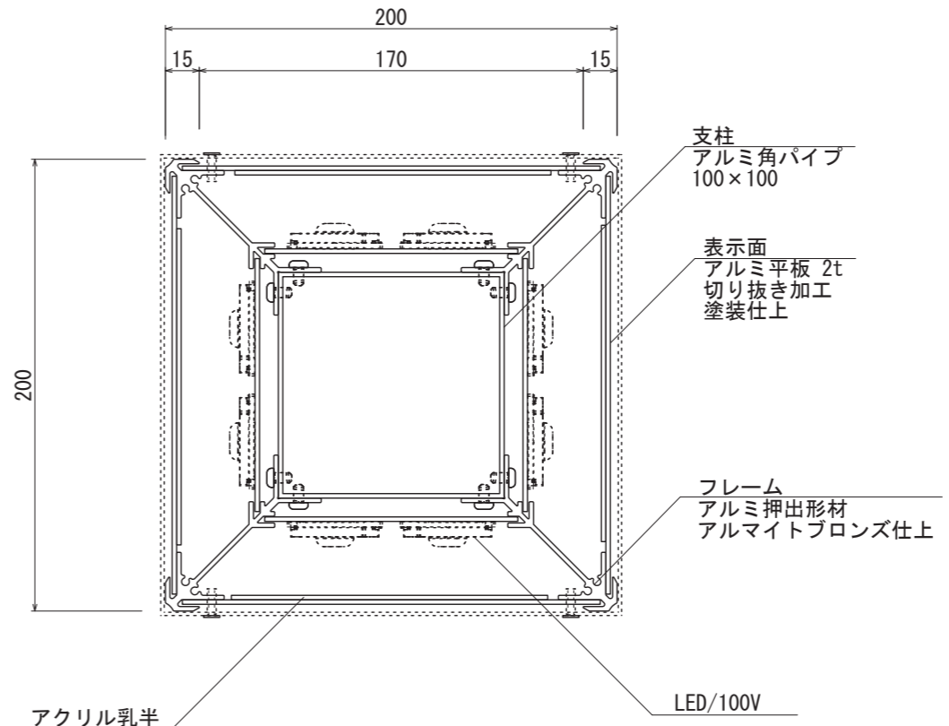
【断面図 S=1:3】
