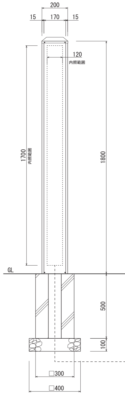
【正面図 S=1:15】
