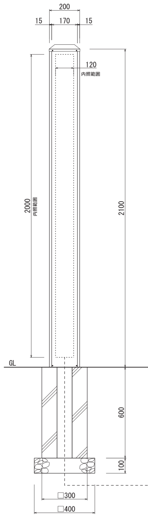
【正面図 S=1:15】
