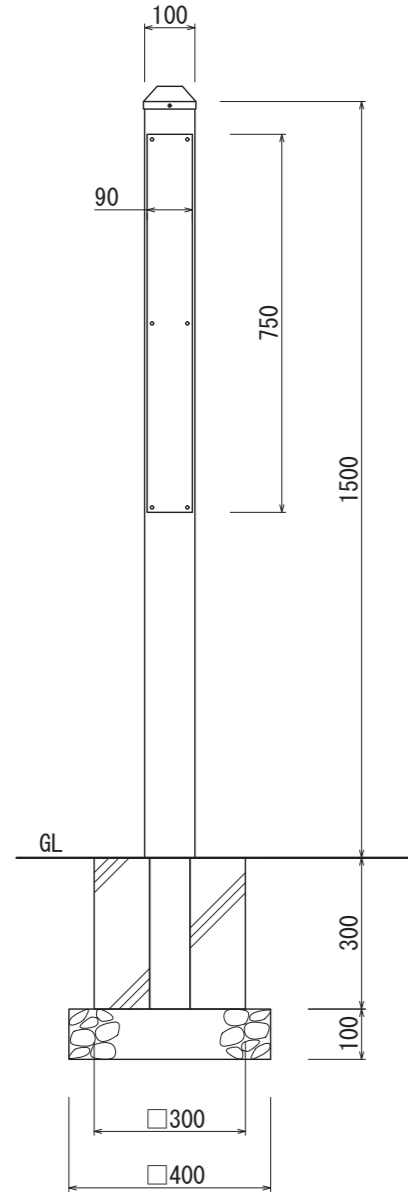
【基礎タイプ】
