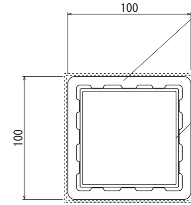
【断面図 S=1:3】
