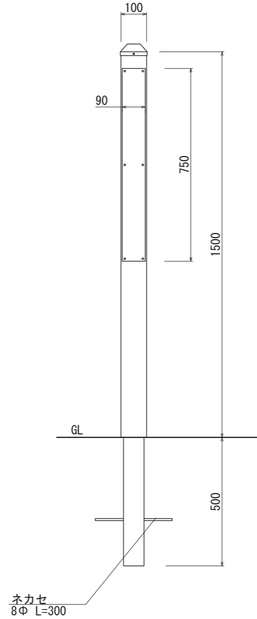
【土中タイプ】
