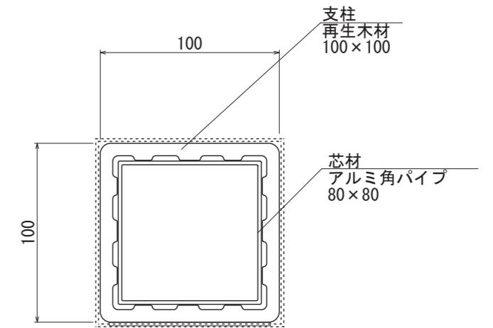
【断面図 S=1:3】
