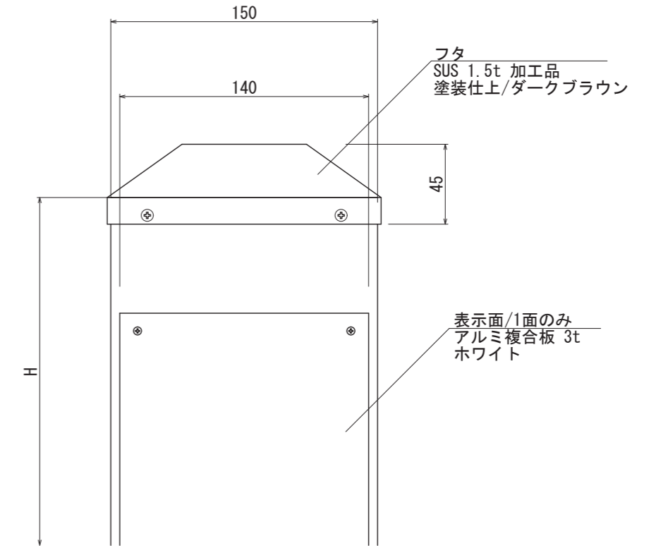
【正面図 S=1:3】
