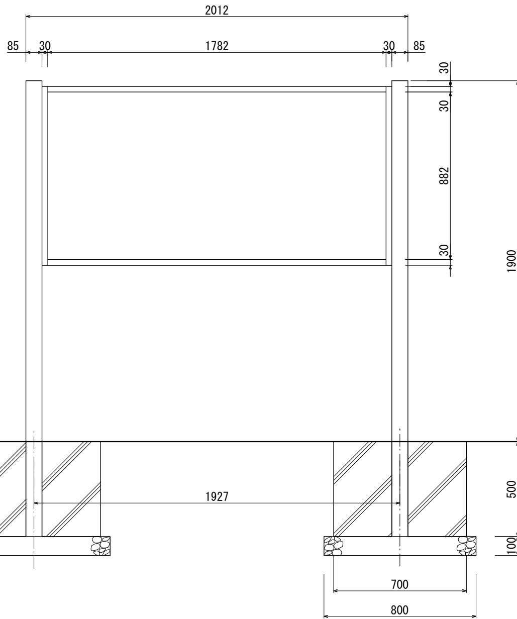
【正面図 S=1:20】
