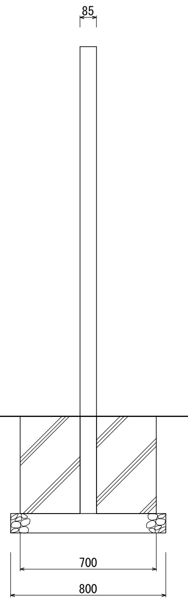
【側面図 S=1:20】
