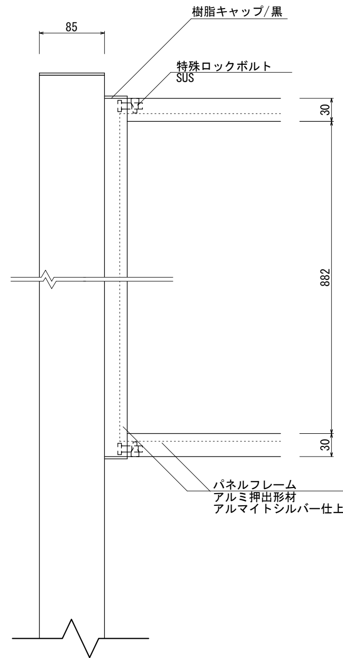
【正面図 S=1:5】
