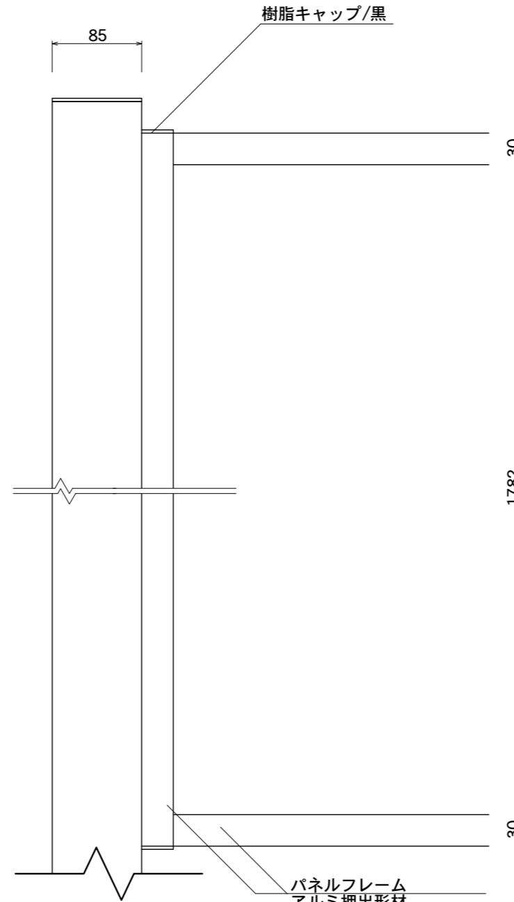
【正面図】
