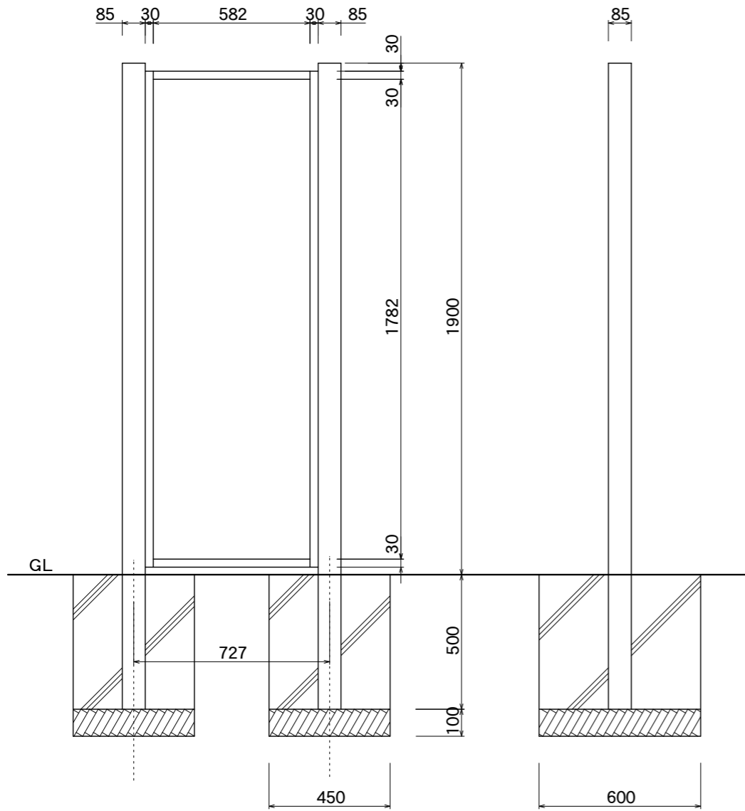
【正面図】
