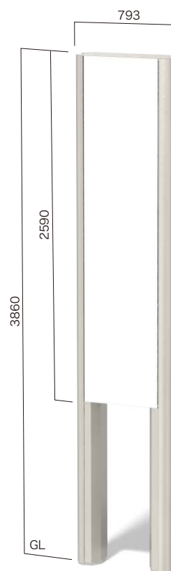
BF-6040A 二本脚 表示有効寸法 W584×H2590両面 設計価格 ¥1,188,000(外税)
