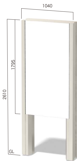
SCP-9026A 二本脚 表示有効寸法 W884×H1795両面 設計価格 ¥1,012,000(外税)
