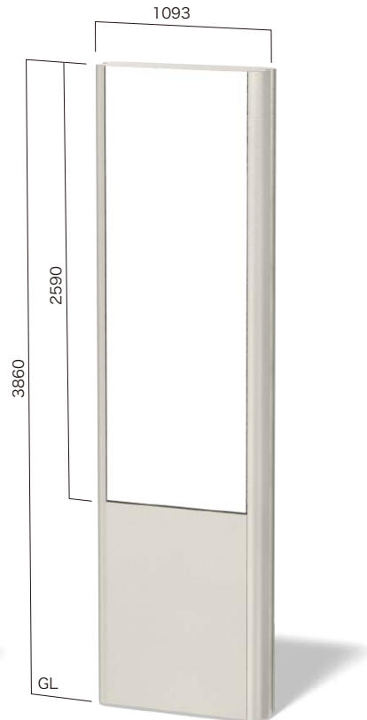
BF-9040K 腰板付 表示有効寸法 W884×H2590両面 設計価格 ¥1,324,000(外税)
