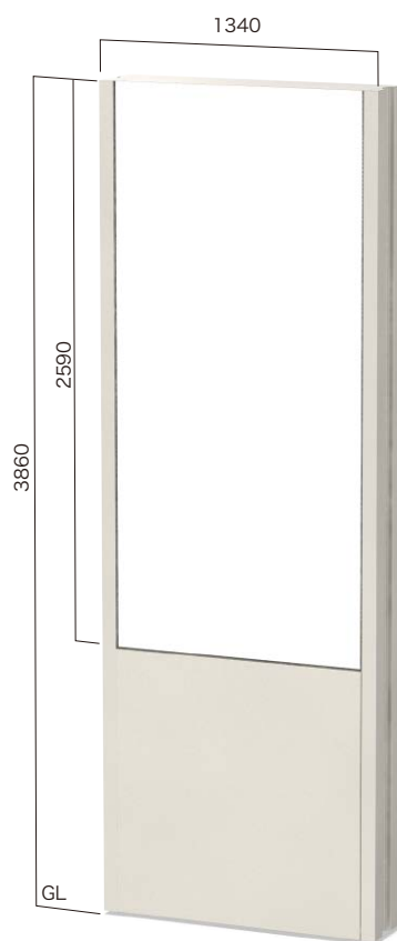
SCP-12040K 腰板付 表示有効寸法 W1184×H2590両面 設計価格 ¥1,570,000(外税)
