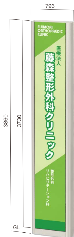
BF-6040F フルフェイス・巾木 表示有効寸法 W584×H3730両面 設計価格 ¥1,268,000(外税)
