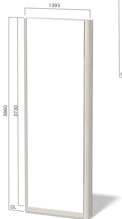
BF-12040F フルフェイス・巾木 表示有効寸法 W1184×H3730両面 設計価格 ¥1,476,000(外税)
