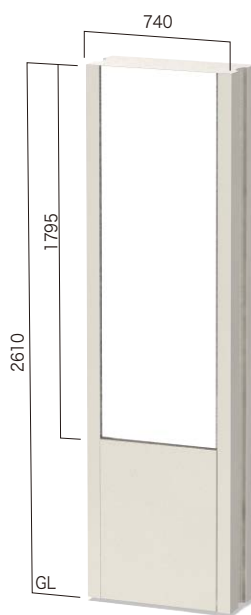
SCP-6026K 腰板付 表示有効寸法 W584×H1795両面 設計価格 ¥948,000(外税)
