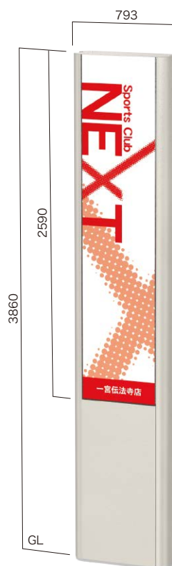
BF-6040K 腰板付 表示有効寸法 W584×H2590両面 設計価格 ¥1,300,000(外税)
