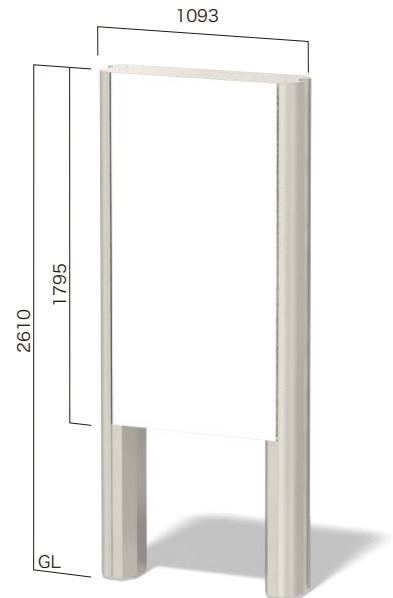
BF-9026A 二本脚 表示有効寸法 W884×H1795両面 設計価格 ¥946,000(外税)
