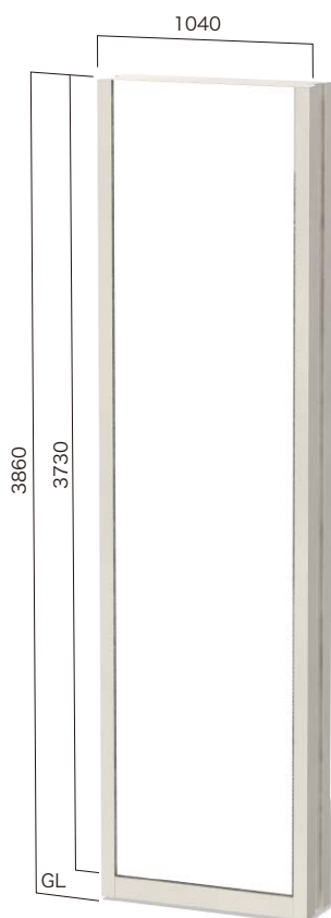
SCP-9040F フルフェイス・巾木 表示有効寸法 W884×H3730両面 設計価格 ¥1,512,000(外税)
