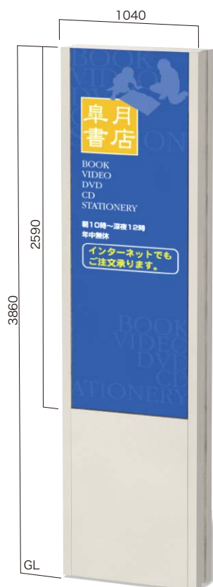
SCP-9040K 腰板付 表示有効寸法 W884×H2590両面 設計価格 ¥1,462,000(外税)
