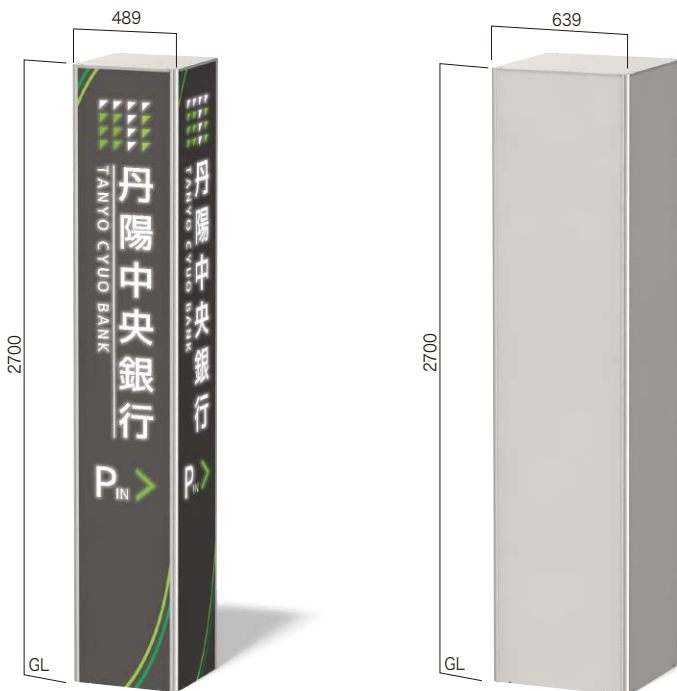
QRX-4527 非内照 表示有効寸法 W423×H2690× 四面 設計価格 ¥543,400( 外税 )
