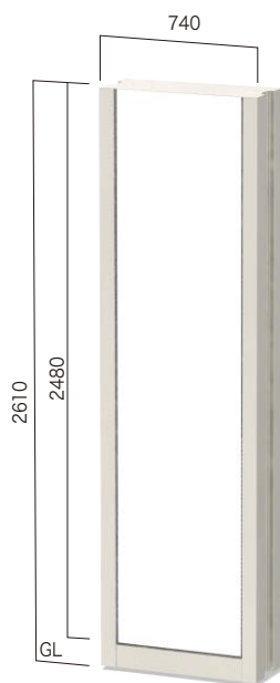
SCP-6026F フルフェイス・巾木 表示有効寸法 W584×H2480両面 設計価格 ¥990,000(外税)
