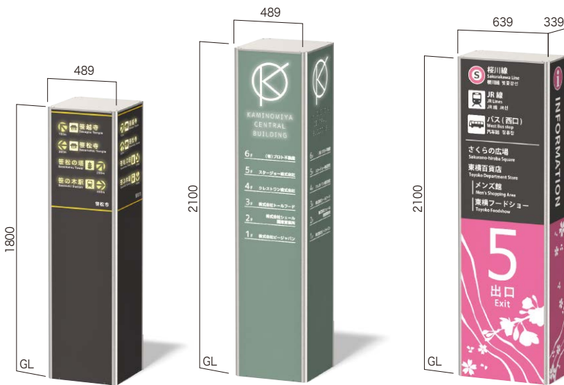
QRX-4518 非内照 表示有効寸法 W423×H1790× 四面 設計価格 ¥349,800( 外税 )
