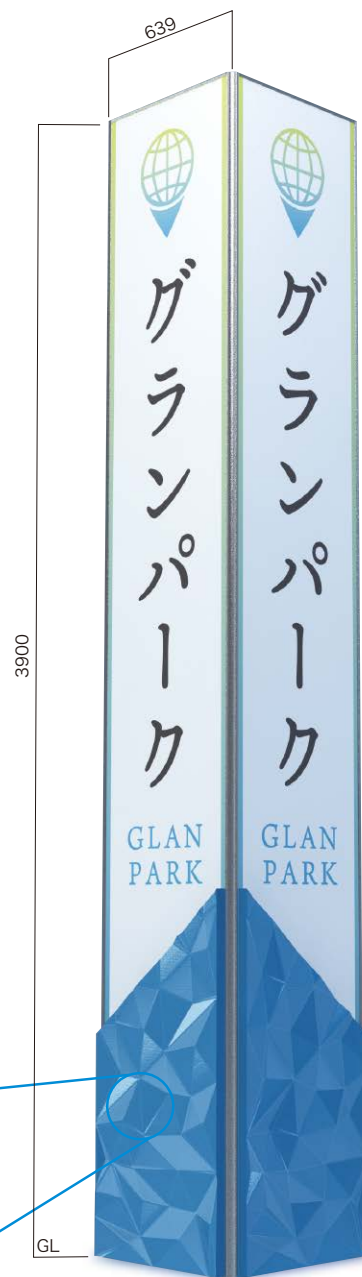
Chic's x クアトロ QRT 表示有効寸法 W573×H3890×四面
