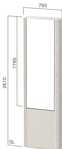
BF-6026K 腰板付 表示有効寸法 W584×H1795両面 設計価格 ¥888,000(外税)
