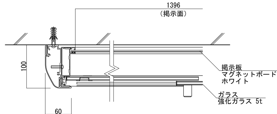
【平面図 S=1:5】
