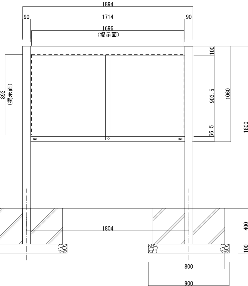
【正面図 S=1:20】
