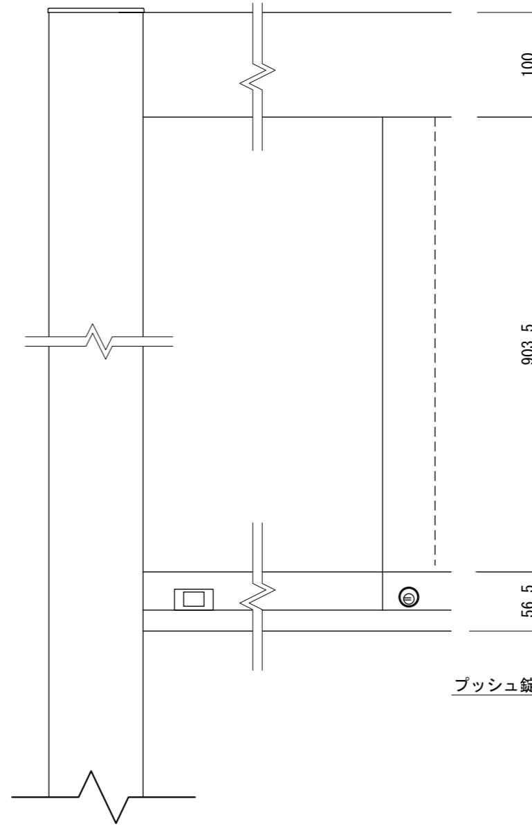
【正面図 S=1:5】
