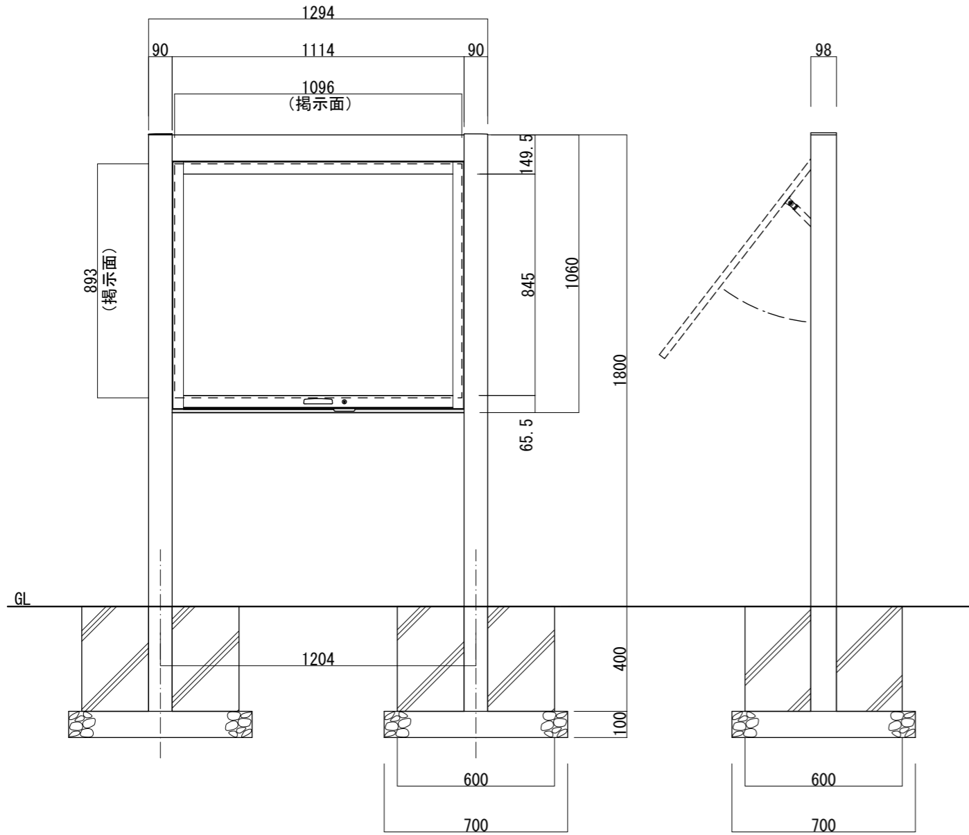
【正面図 S=1:20】
