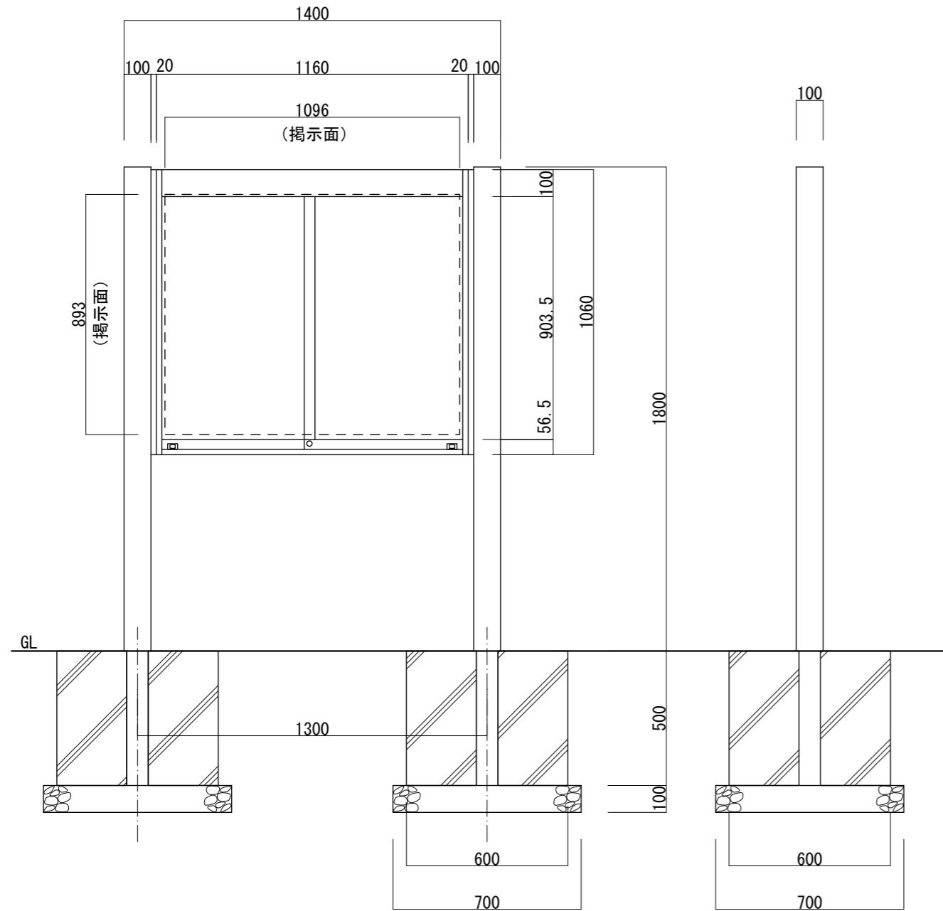
【正面図 S=1:20】
