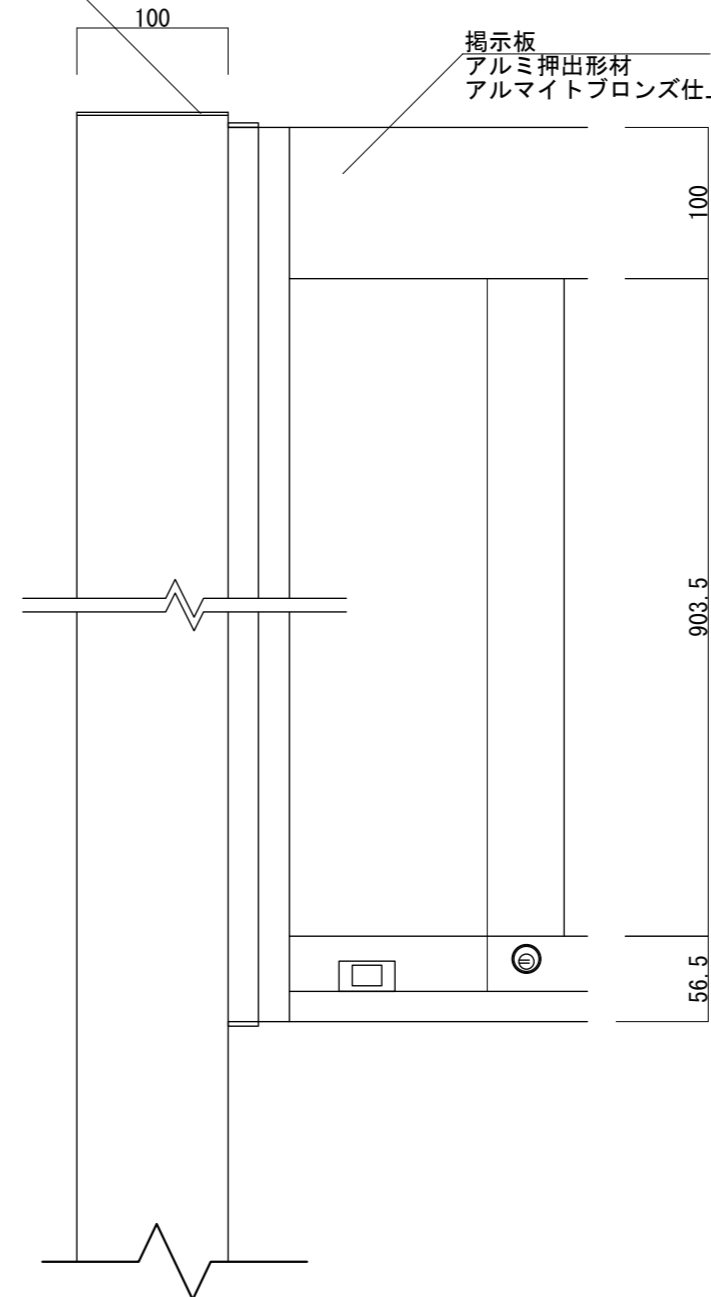
【正面図 S=1:5】
