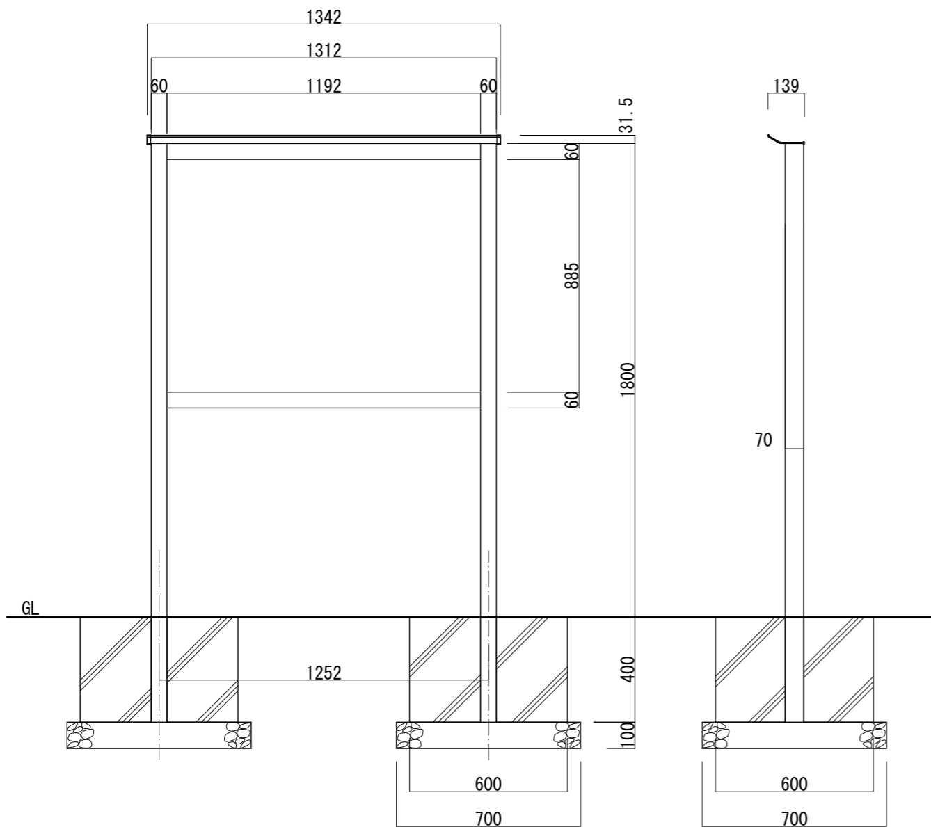
【正面図 S=1:20】
