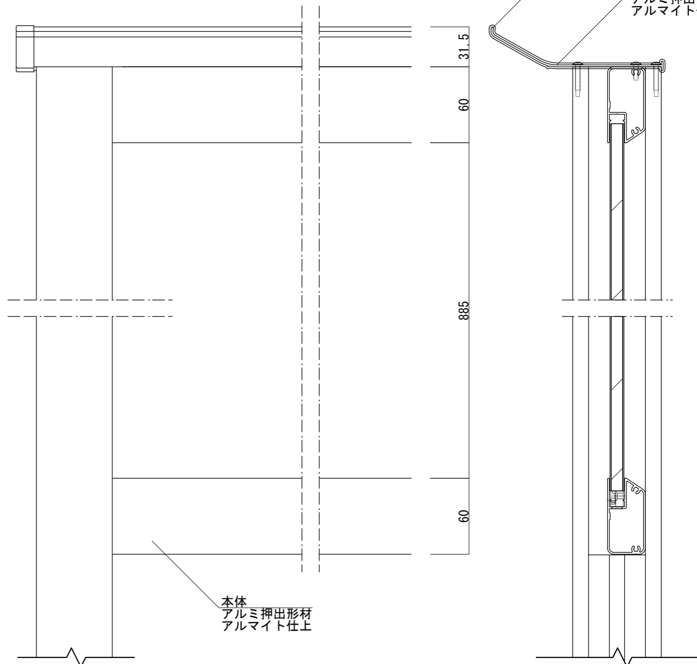
【正面図 S=1:3】
