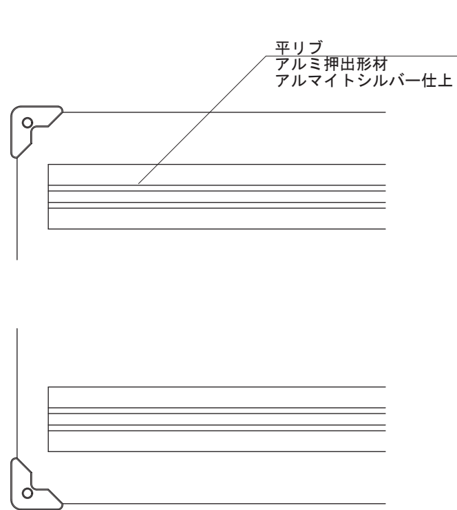
【背面図 S=1:5】
