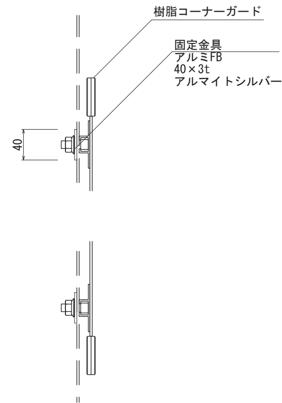
【側面図 S=1:5】
