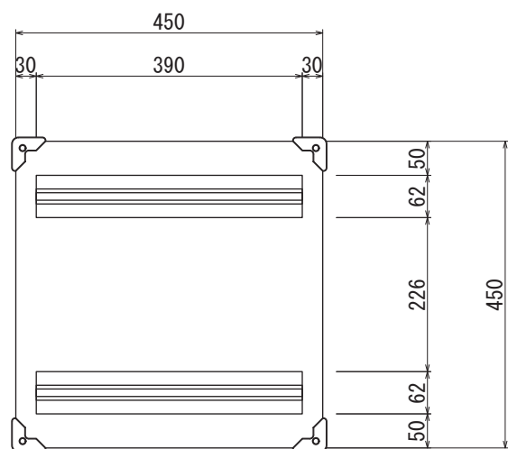
【背面図 S=1:10】
