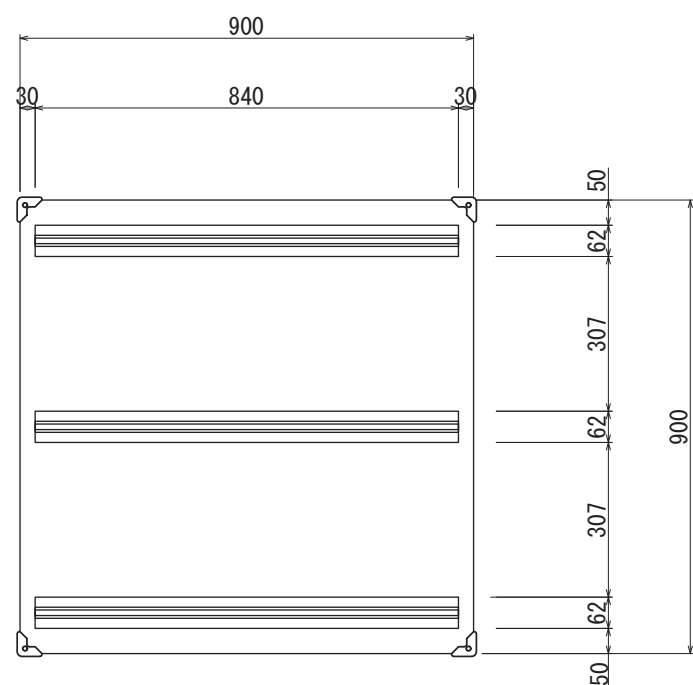
【背面図 S=1:15】
