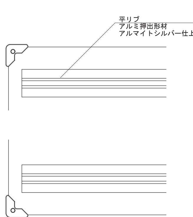
【背面図 S=1:5】
