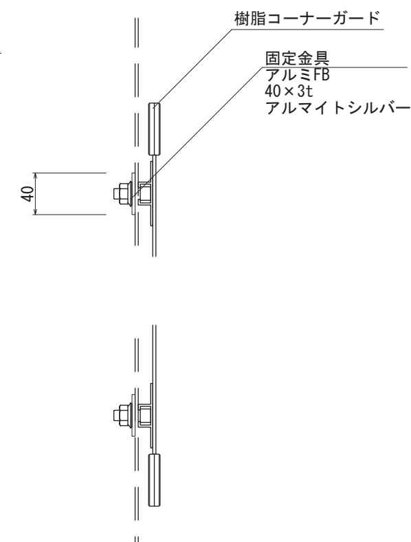
【側面図 S=1:5】
