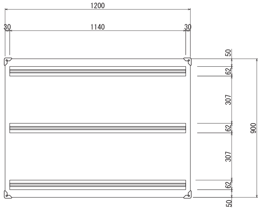
【背面図 S=1:15】
