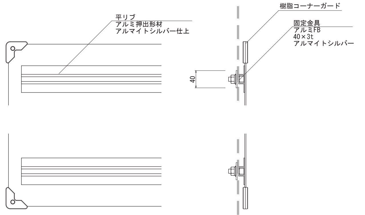
【背面図 S=1:5】
