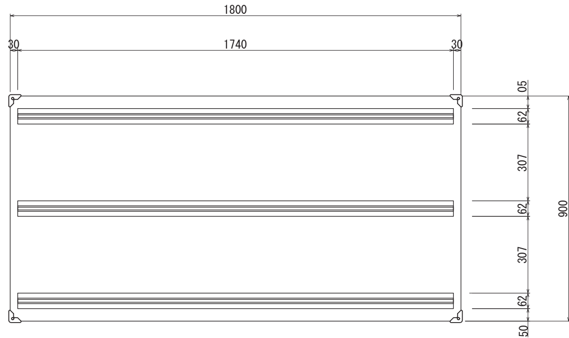
【背面図 S=1:15】
