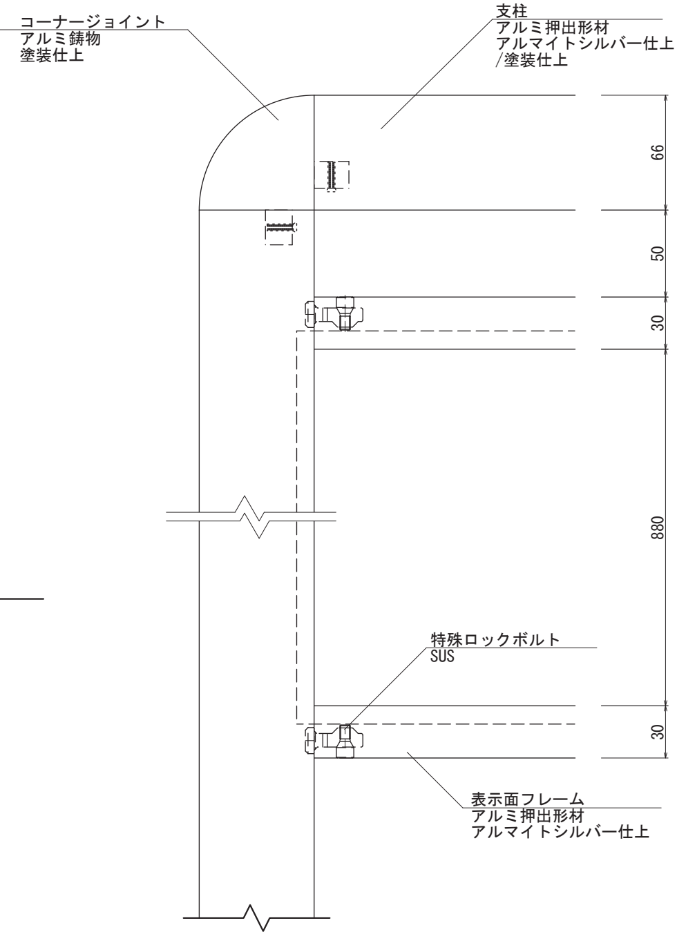
【正面図 S=1:3】
