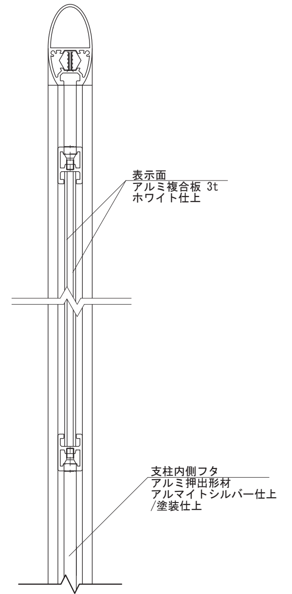
【側面図 S=1:3】
