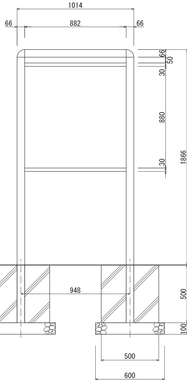
【正面図 S=1:20】
