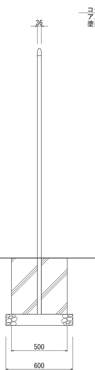
【側面図 S=1:20】
