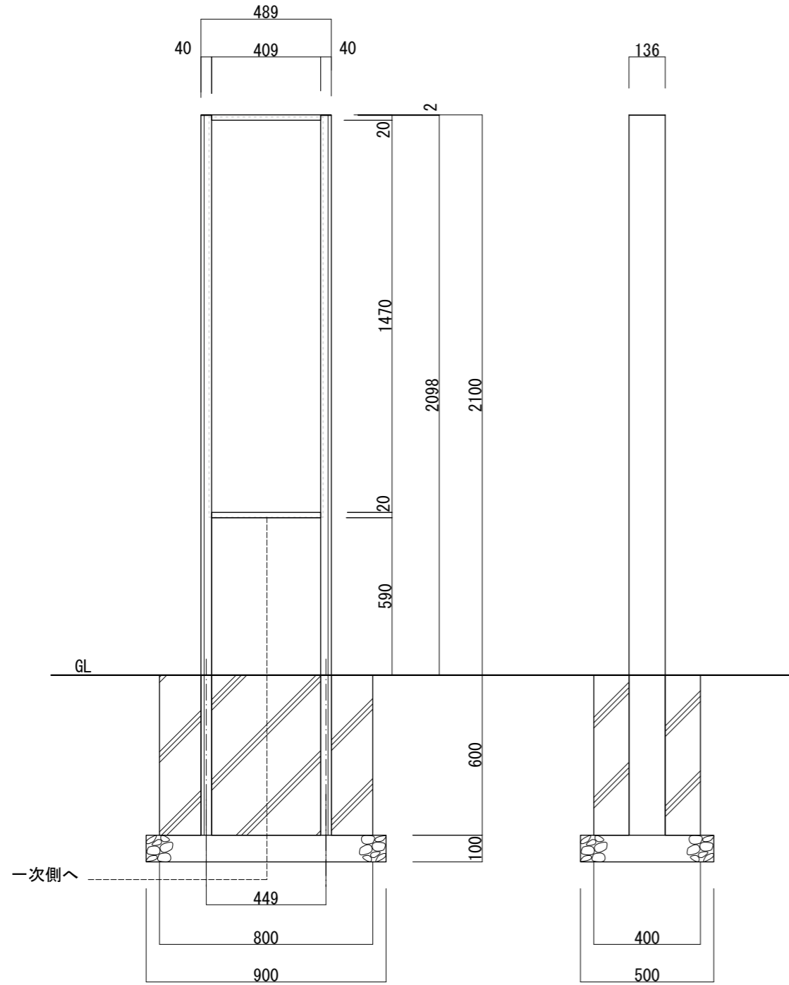
【正面図 S=1:20】
