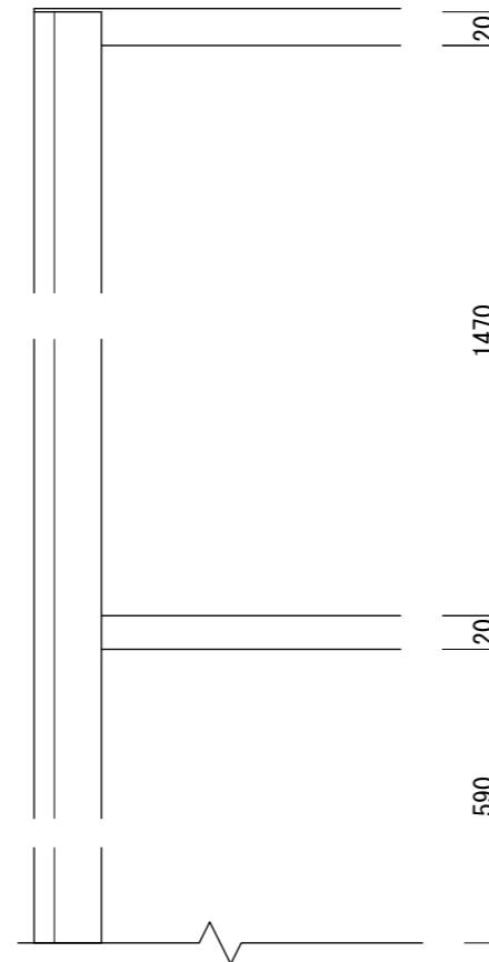
【正面図 S=1:5】
