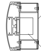
【A-A断面図 S=1:5】
