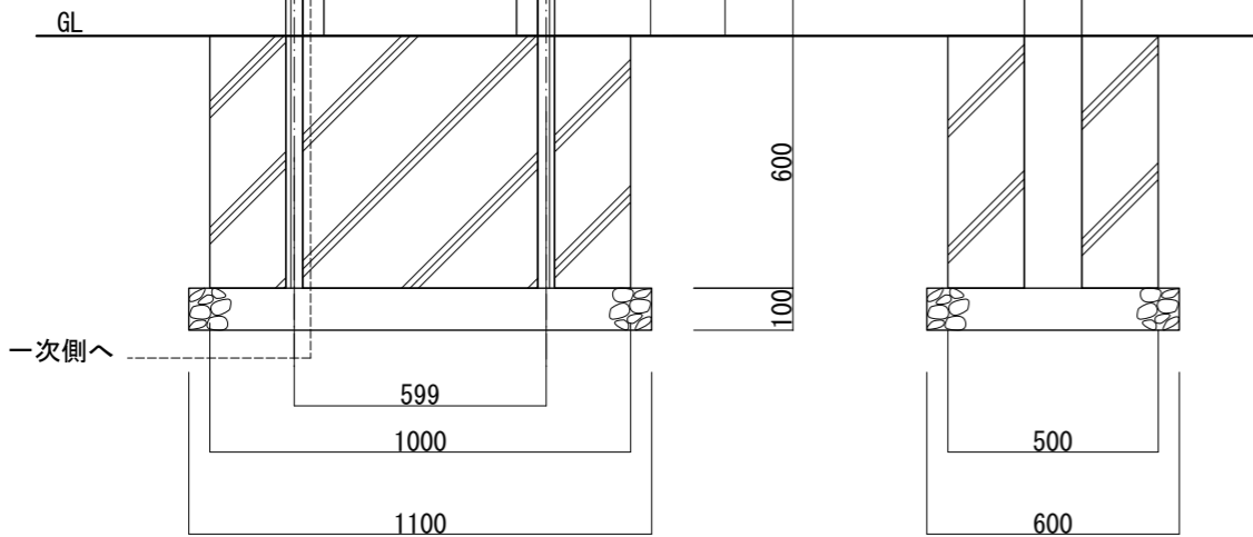
【正面図 S=1:20】
