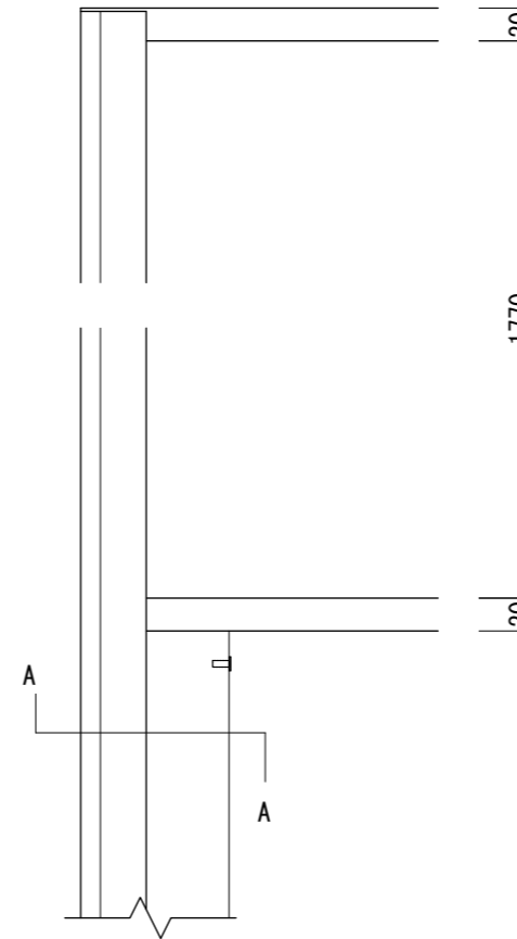
【正面図 S=1:5】
