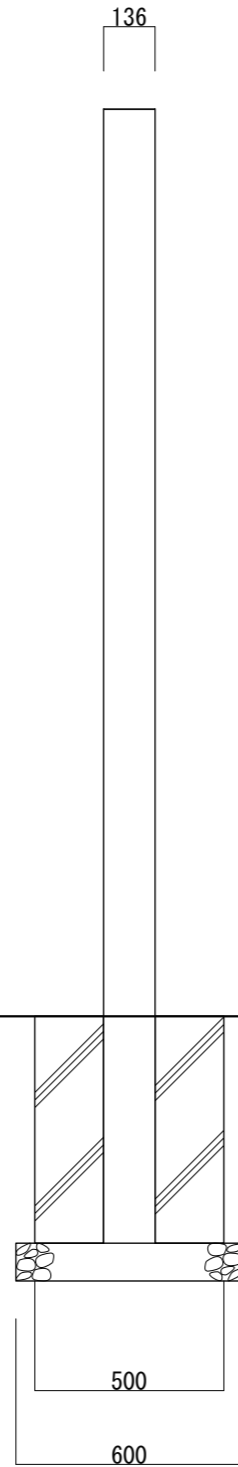
【側面図 S=1:20】
