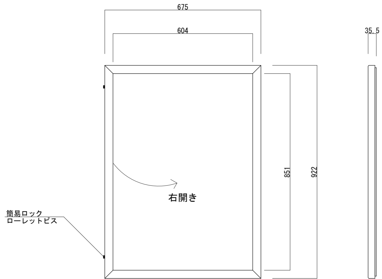
【正面図 S=1:10】
