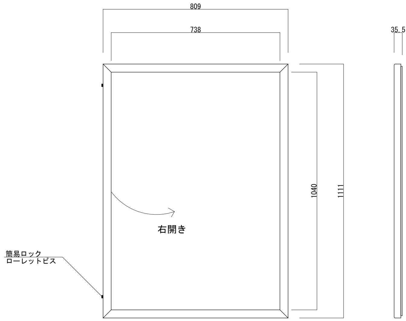
【正面図 S=1:10】
