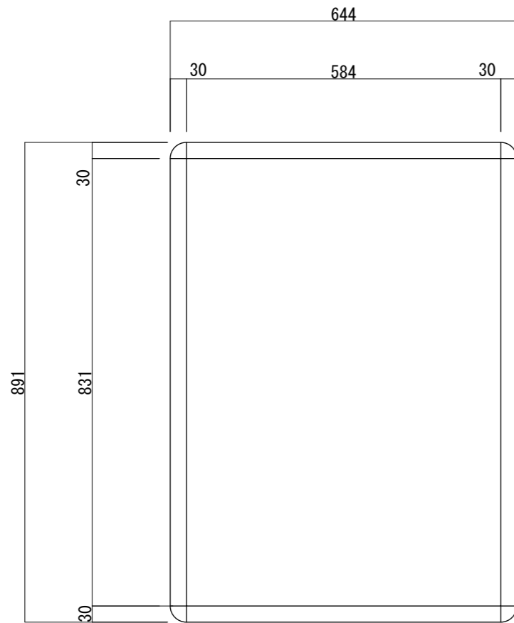
【正面図 S=1:10】
