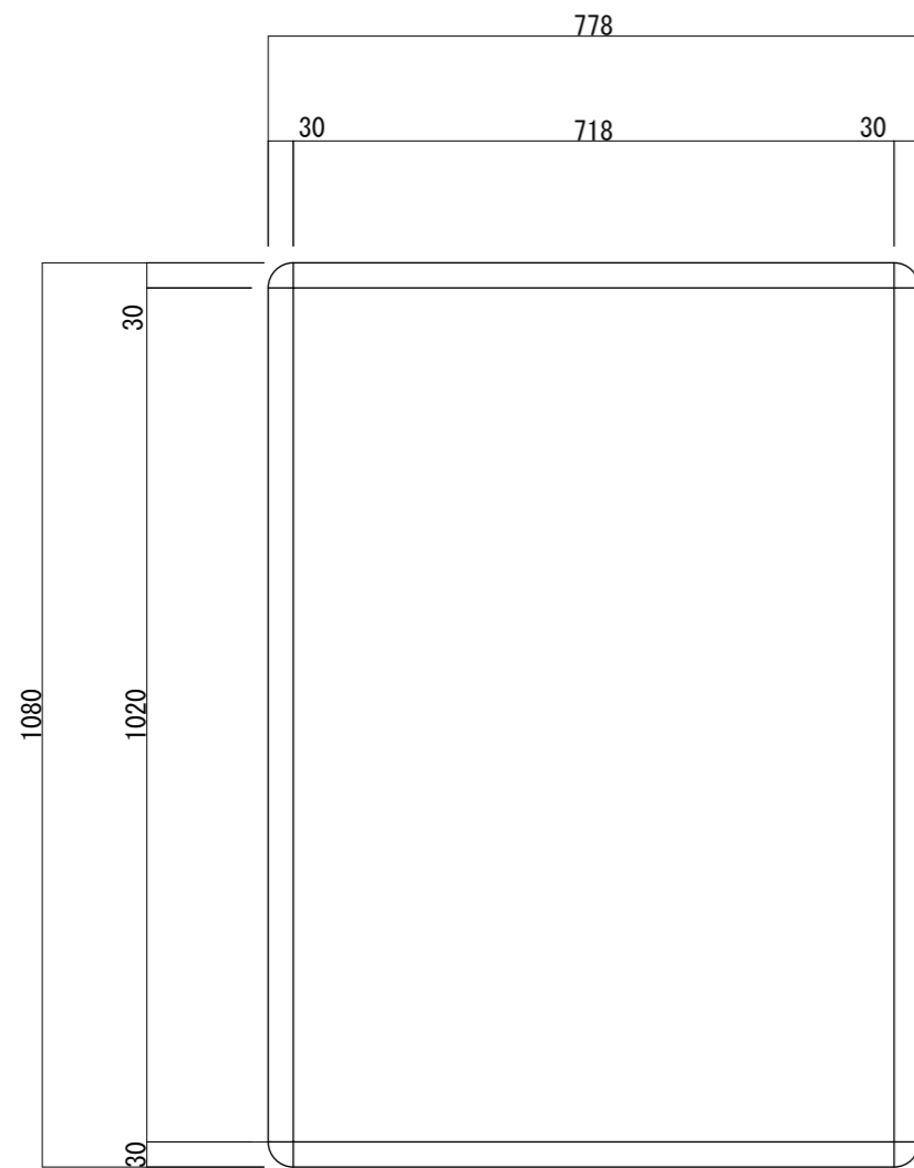
【正面図 S=1:10】
