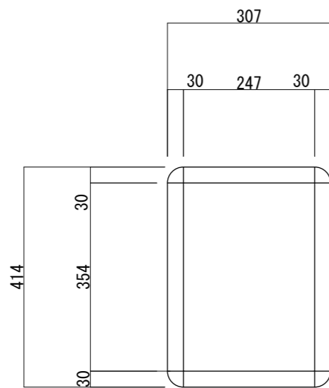
【正面図 S=1:10】
