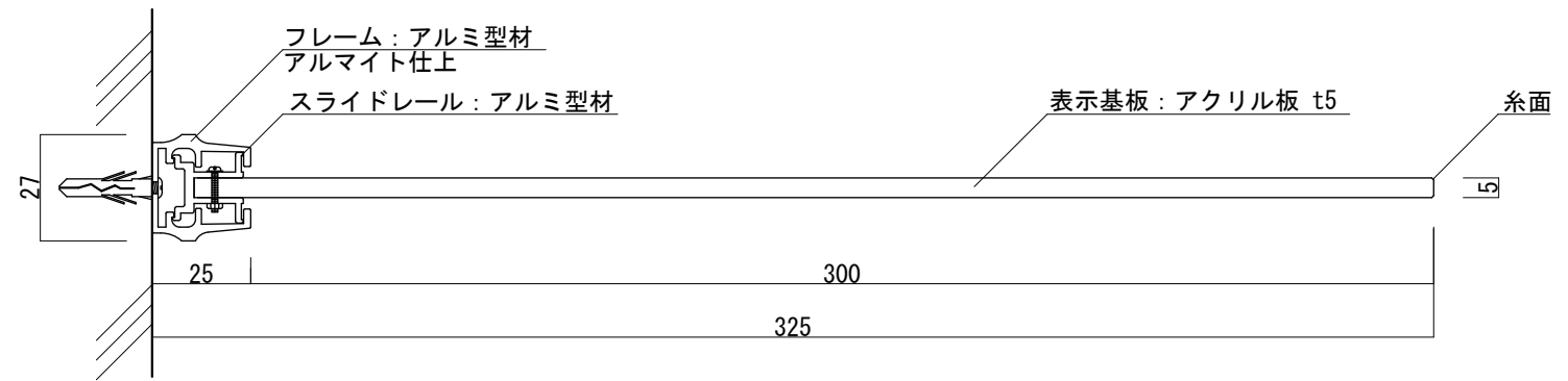
【平面図 S=1:2】
